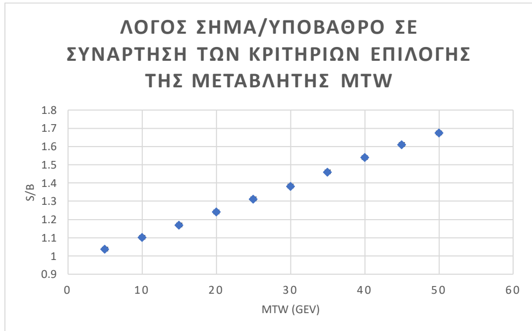
Εικόνα 5.20: Διάγραμμα του λόγου S/B σε συνάρτηση με τα κριτήρια επιλογής της μεταβλητής mtw.
