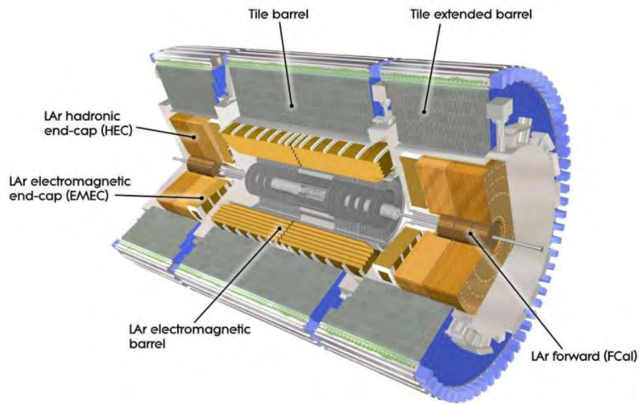
Εικόνα 4.11: Αποκομμένη όψη του συστήματος θερμιδόμετρου ATLAS[56].
