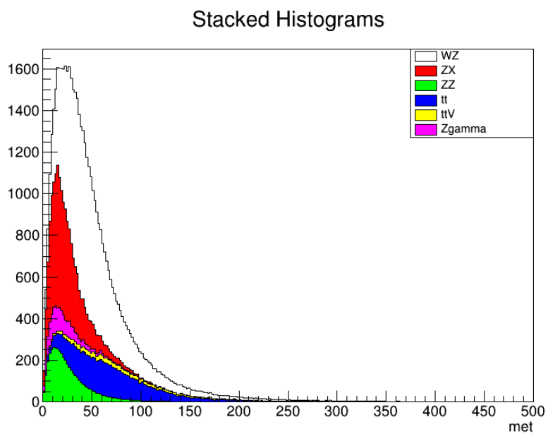
Εικόνα 5.10: Ιστόγραμμα με τη μεταβλητή της ελλείπουσας εγκάρσιας ενέργειας.
