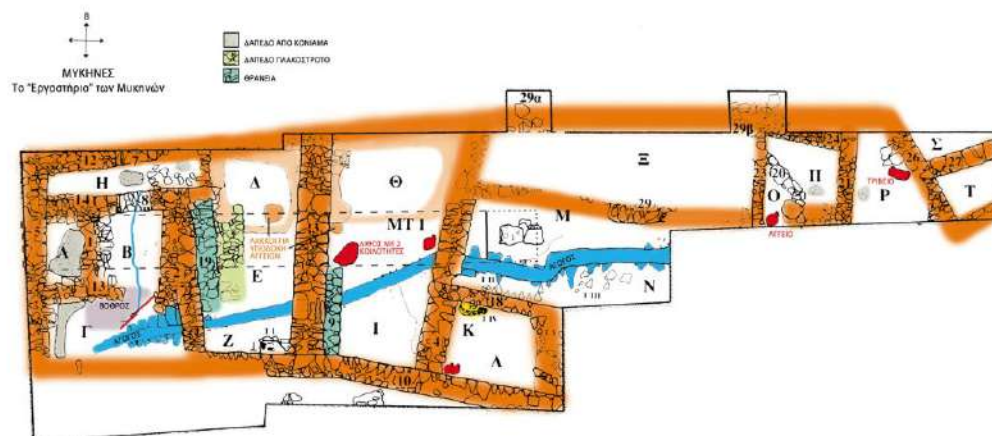
Εικ 7. Αρχιτεκτονική κάτοψη του Εργαστηρίου των Μυκηνών (Παϊπέτη 2019, Α-6)
