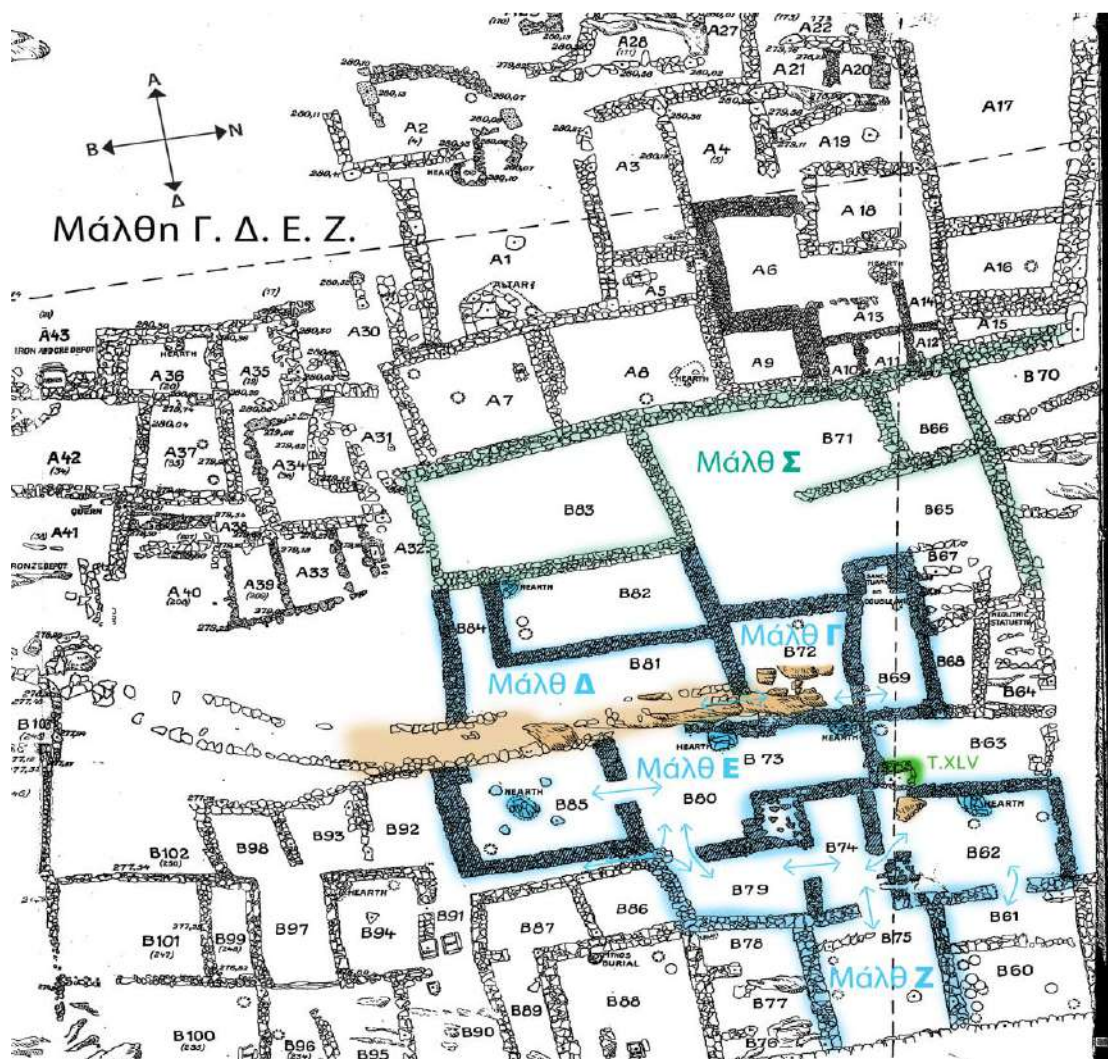
Εικ. 42. Κάτοψη οικίας Κ Μάλθης (Παϊπέτη 2019, Α- 38)
