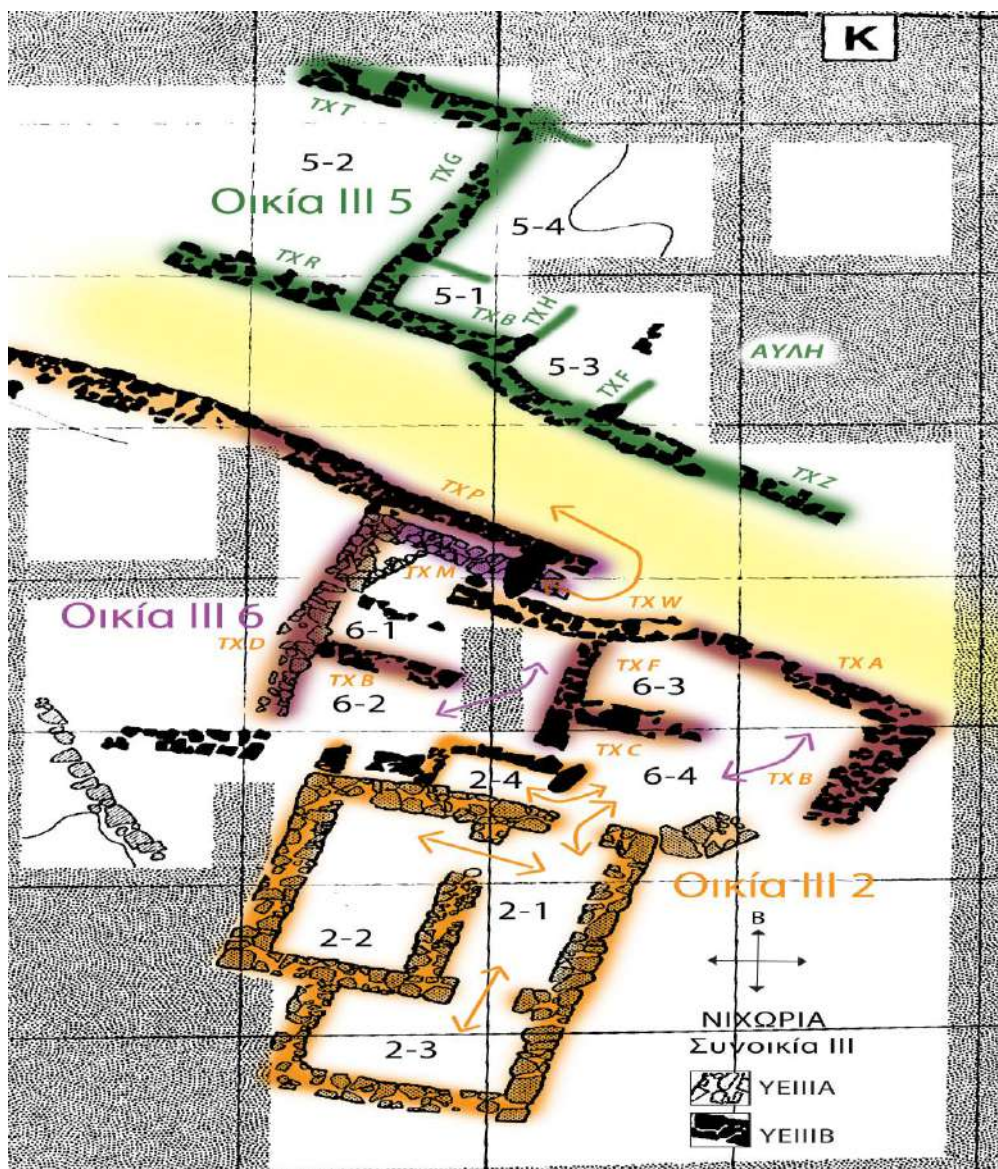
Εικ.30. Συνοικία III Νιχώρια (Παϊπέτη 2019, Α-31)
