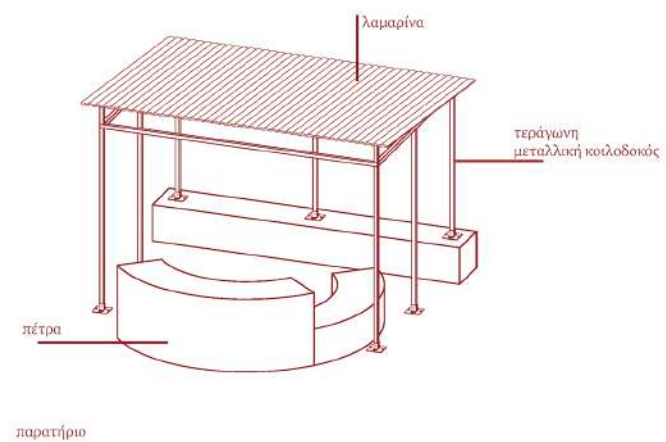
στοιχεία κατασκευής
