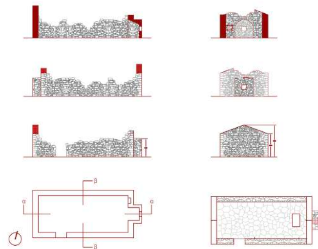
αποτύπωση εκκλησίας ψηλού Αϊ Γιάννη
