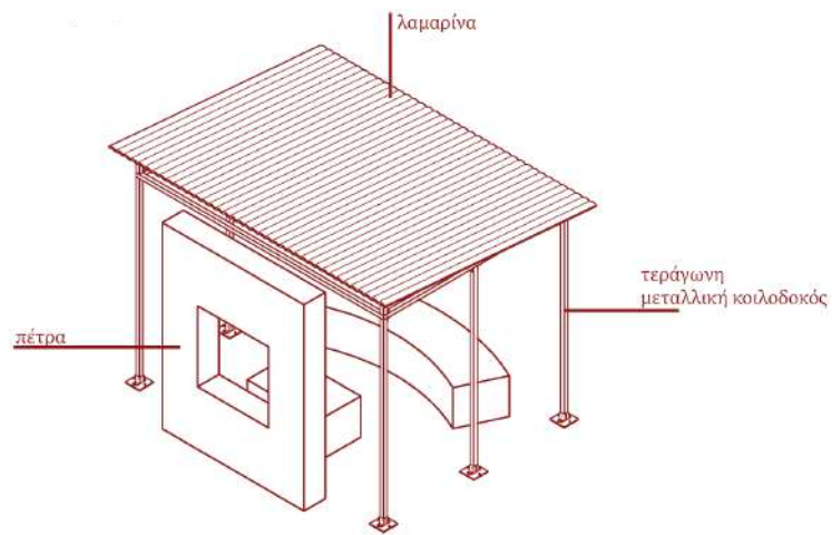
στοιχεία κατασκευής
