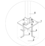
5. βάση στήριξης μόνιμων κατασκευών
