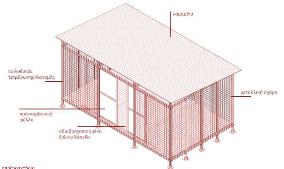
αποξηραντήριο
