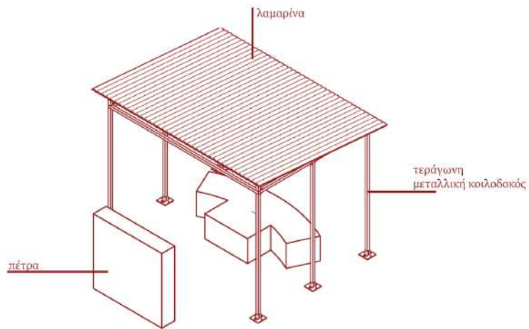
στοιχεία κατασκευής
