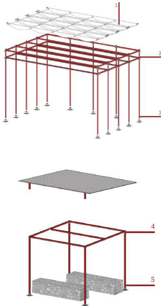
2. μηχανισμός αρθρωτής σκαλωσιάς
