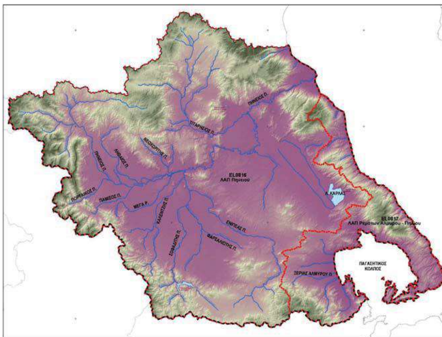
Εικόνα 6: Λεκάνες απορροής ποταμού στο Υ.Δ. Θεσσαλίας (EL08) και κυριότερα ποτάμια και λίμνες. Πηγή: ΥΠΕΝ, 2020
