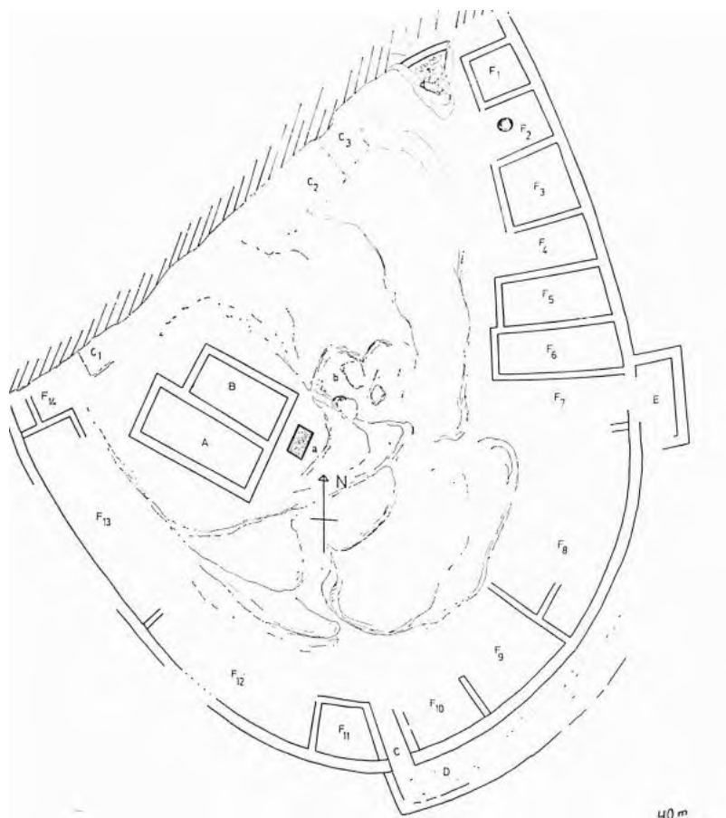
Εικόνα 28. Ακρόπολη Λαθούριζας (46°). Κάτοψη (Lauter-Bufe 1979, σχεδ. 2)
