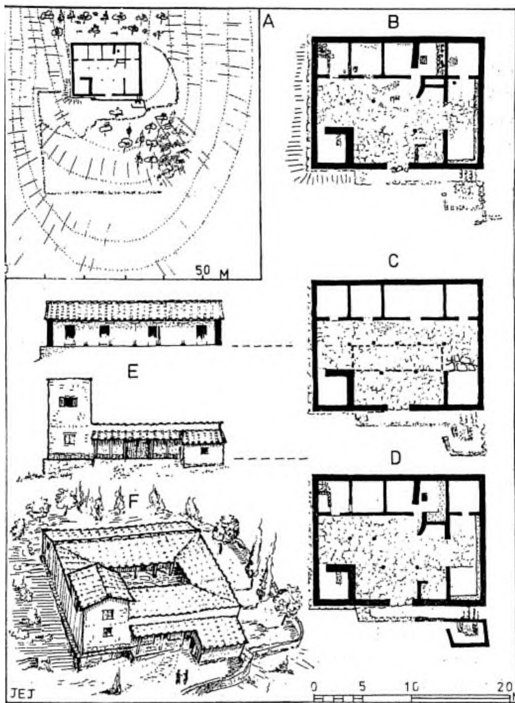
Εικόνα 23. Οικία της Βάρης: Α: κάτοψη. Β-С-Д: οικοδομικές φάσεις. Ε-Ε: σχεδιαστική αποκατάσταση της οικίας (Jones 1975, 115, εικ.17)
