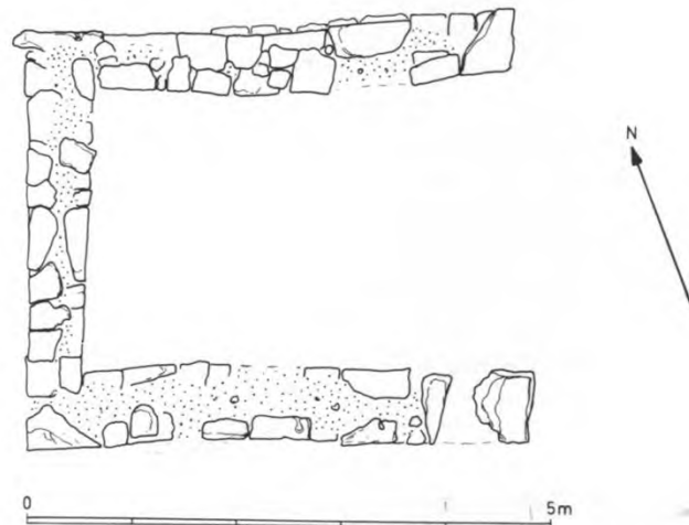
Εικόνα 64. Κάτοψη του Ναϊσκού στη βόρεια πλευρά της Λαθούριζας (Lauter 1985, σχεδ.8)
