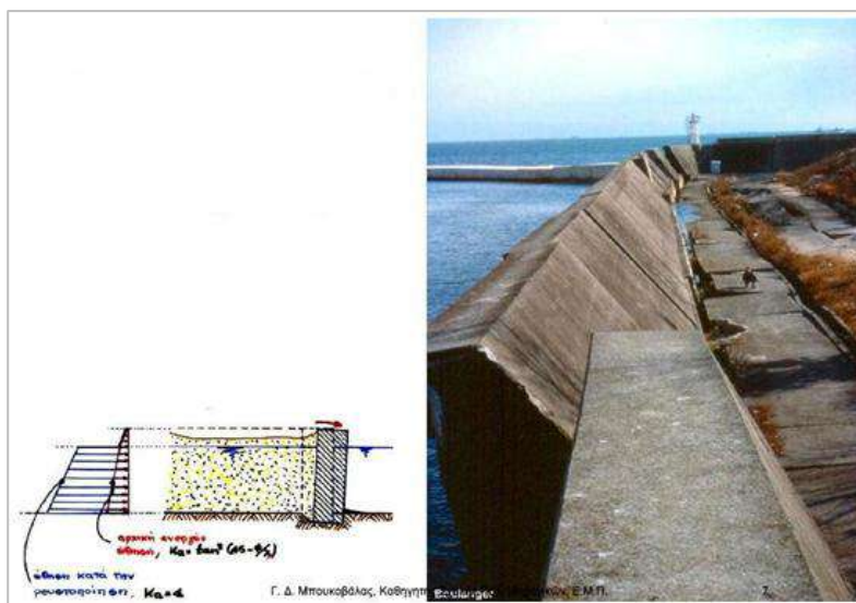
Εικόνα 13: Στοχία σε λιμενικούς κρηπιδότοιχους - Kobe, Ιαπωνία (1995)
