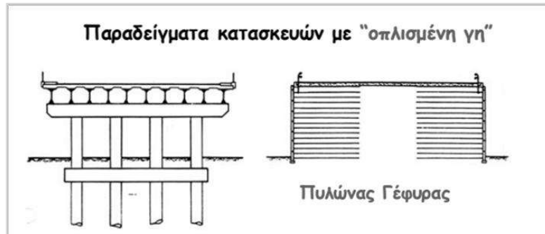
Παραδείγματα κατασκευών με «οπλισμένη γη» - Πυλώνας Γέφυρας. Πηγή: Μπουκοβάλας, 2009
