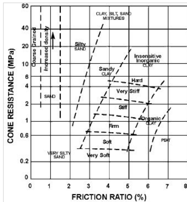
Εικόνα 26: Κατάταξη εδάφους από δεδομένα CPT σύμφωνα με Meigh (1987)
