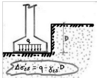
Σχήμα 9: Αύξηση βάθους θεμελίωσης "επιπέουσα" θεμελίωση. Πηγή: Μπουκοβάλας, 2009
