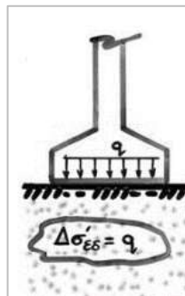
Σχήμα 8: Αύξηση βάθους θεμελίωσης "επιπέουσα" θεμελίωση. Πηγή: Μπουκοβάλας, 2009
