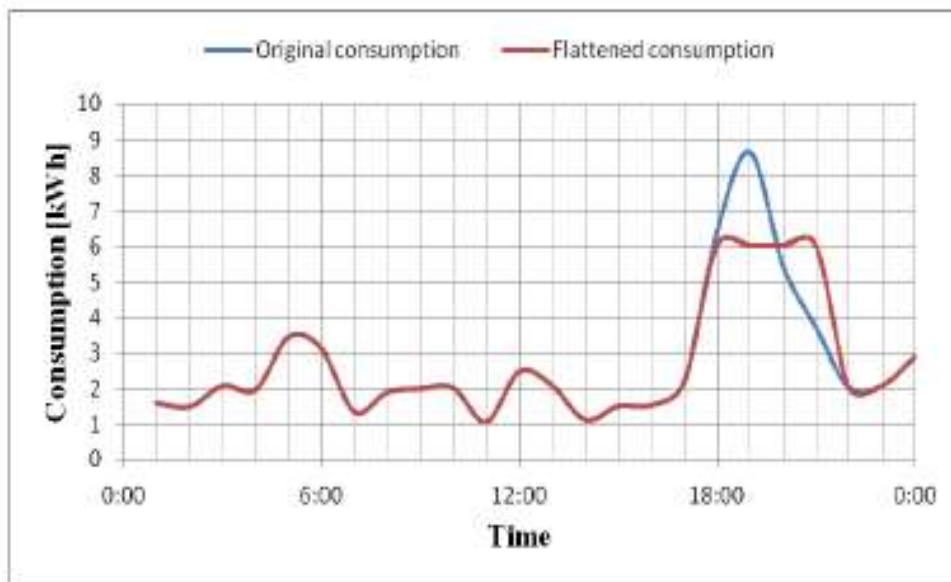
Εικόνα 6.30: Κατανάλωση νοικοκυριού 5 στις 25 Απριλίου
