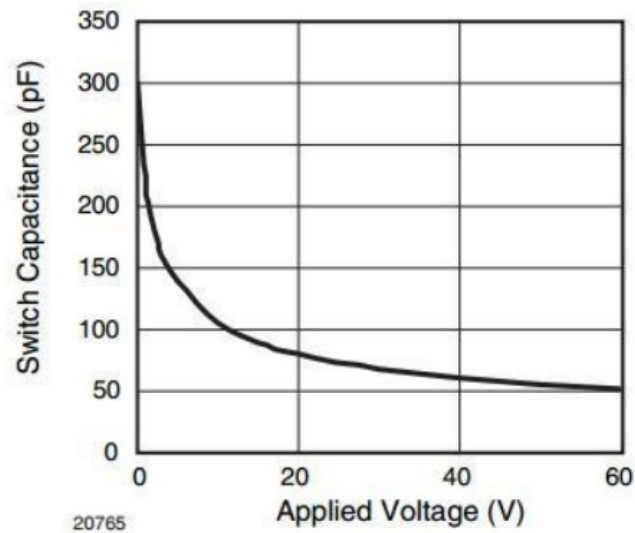
Εικόνα 3.2: Χωρητικότητα διακόπτη σε σχέση με την εφαρμοζόμενη τάση (research gate.net)
