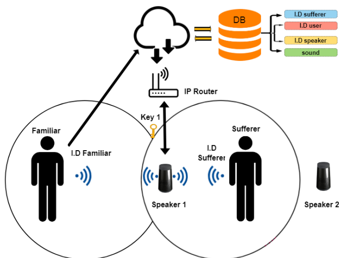
Σχήμα 4.2: Αναπαράσταση της αρχιτεκτονικής του προτεινόμενου συστήματος στο επίπεδο της επικοινωνίας του χρήστη.
