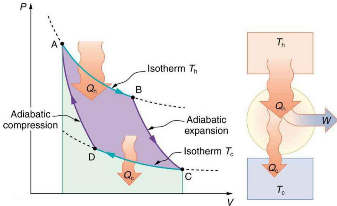
Εικόνα 1.2 Κύκλος Carnot.
