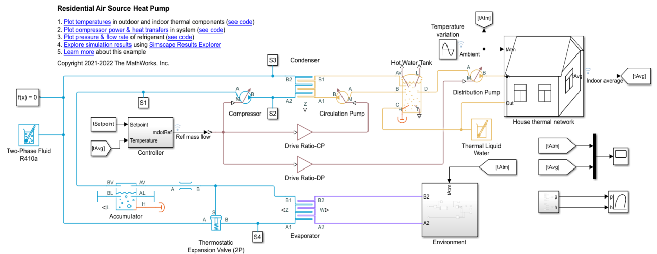
Εικόνα 4.1 Περιβάλλον μοντέλου στο Simulink.
