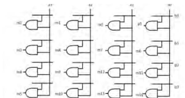
Εικόνα 1.13 Παραγωγή μερικών γινομένων με χρήση πυλών AND
