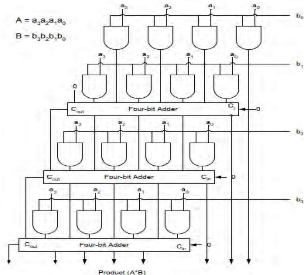
Εικόνα 1.10 Δομή λογικών πυλών αλγορίθμου πολλαπλασιασμού πίνακα για 4x4 bits
