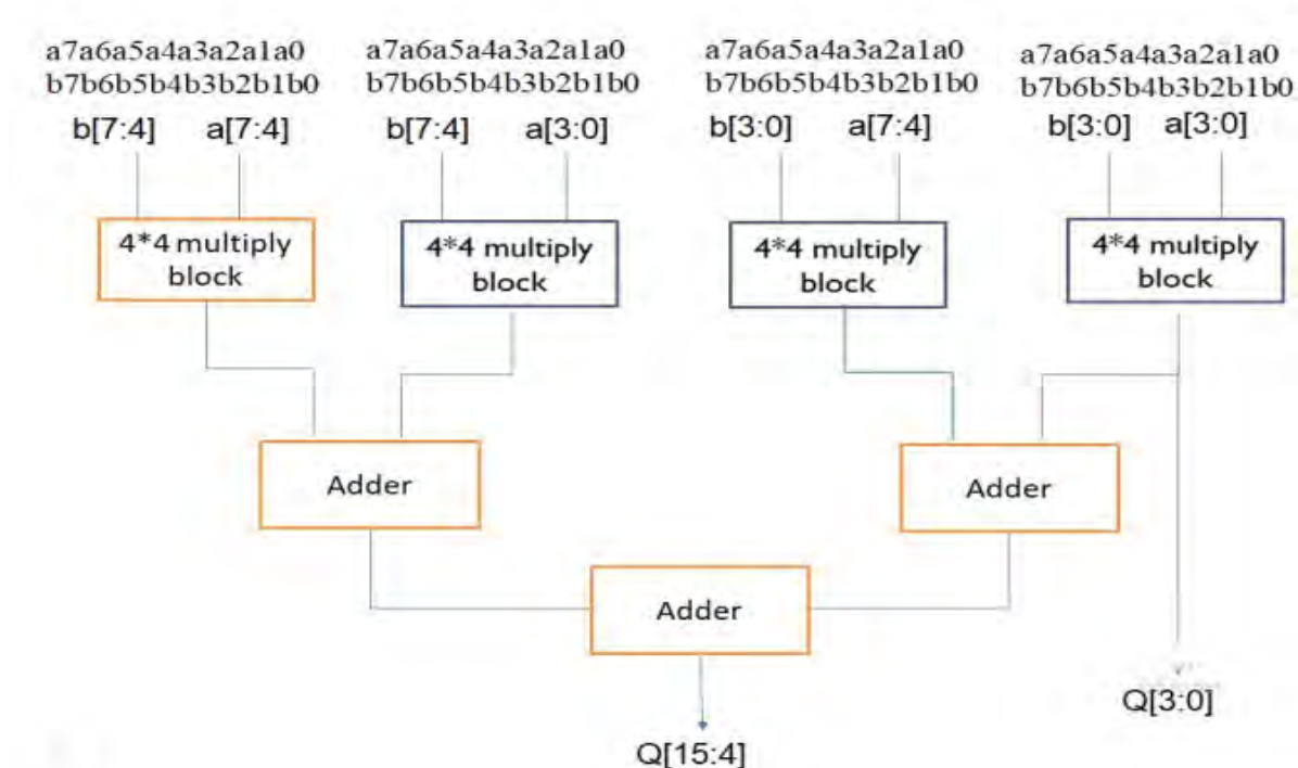
Εικόνα 1.4 Αλγόριθμος πολλαπλασιασμού Vedic για 8x8 bits
