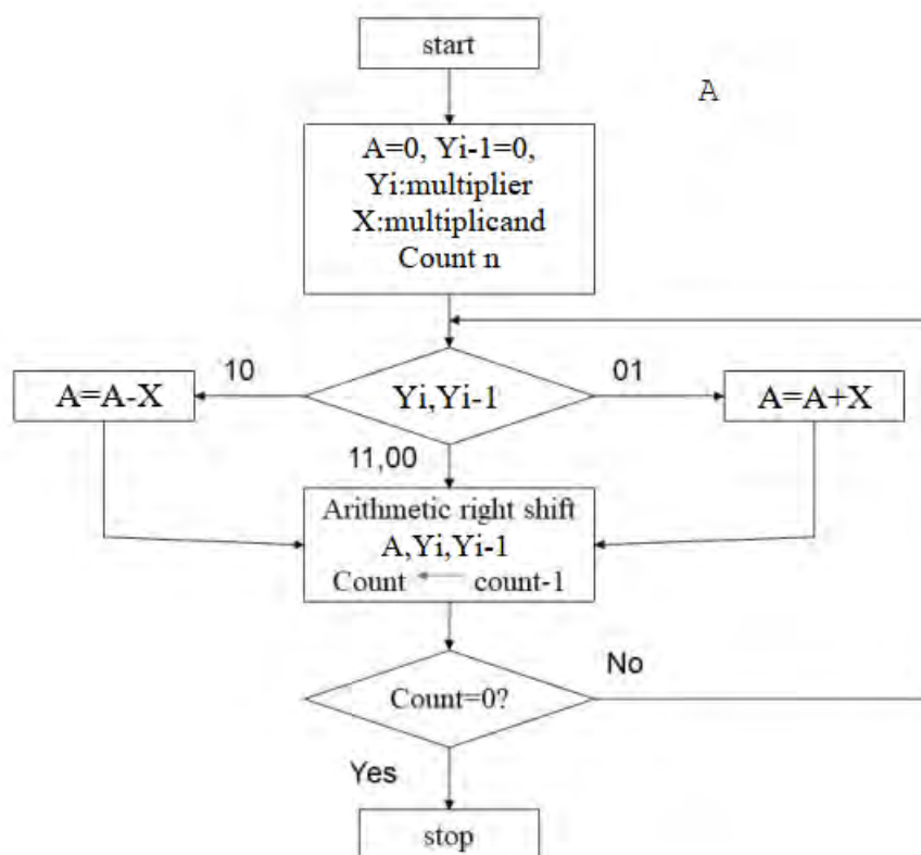
Εικόνα 1.1 Λογικό διάγραμμα αλγόριθμου πολλαπλασιασμού Booth
