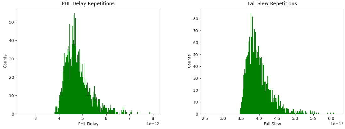
(a) 4 INVx13 PHL Delay
