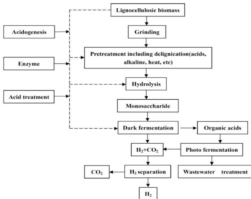
Εικόνα 2: Ένα σχηματικό διάγραμμα για την παραγωγή βιοϋδρογόνου από υλικά λιγνοκυτταρίνης
