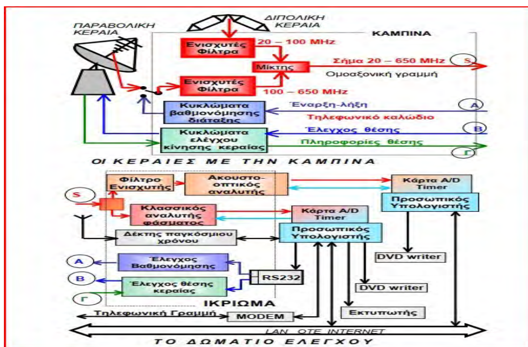
Εικόνα 1.5. Συνοπτικό διάγραμμα δομικής σύστασης του ηλιακού ραδιοφασματογράφου ARTEMIS IV /JLS. [2]
