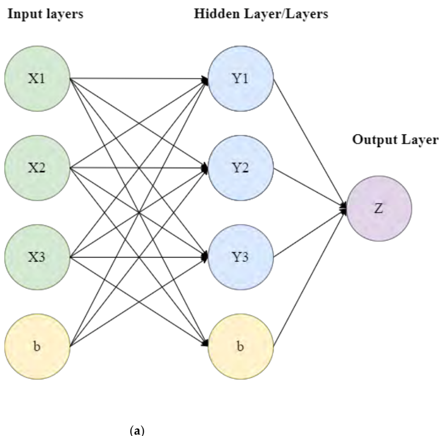
Σχήμα 4. Σχηματική αναπαράσταση της λειτουργίας και αρχιτεκτονικής ενός ANN. Η “input layer” (X) τροφοδοτεί μαζί με το bias της τις κρυφές “hidden layers” (y) οι οποίες παράγουν αποτέλεσμα, εφαρμόζεται σε αυτές η συνάρτηση ενεργοποίησης (εδώ σιγμοειδής) και διαδοχικά τροφοδοτούν τις επόμενες layers η κάθε μία μέχρι την τελική “output layer”.
