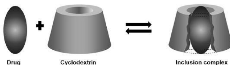
Εικόνα 2.1.3: Δημιουργία συμπλόκου εγκλεισμού
