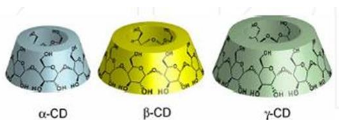
Εικόνα 2.1.1: Απεικόνιση των τριών τύπων κυκλοδεξτρινών (Szejtli, 2004)
