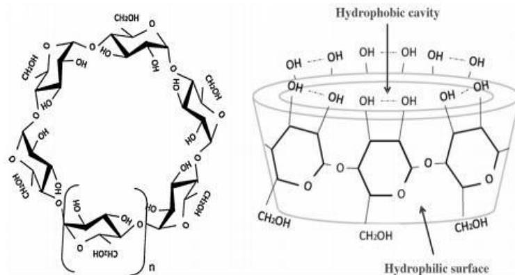
Εικόνα 2.1.2: Αριστερά: Χημική δομή γλυκοζιτικής μονάδας, Δεξιά: Σχήμα κόλουρου κώνου των κυκλοδεξτρινών (Munin and Edwards, 2011)
