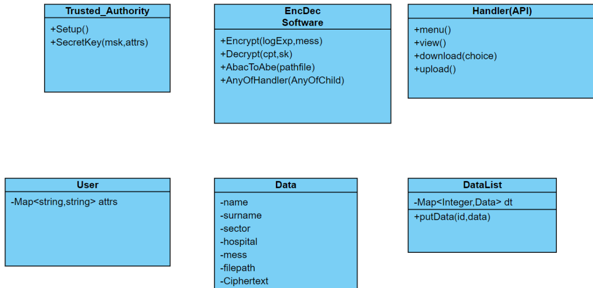
Εικόνα 5.1 Διάγραμμα Κλάσεων
