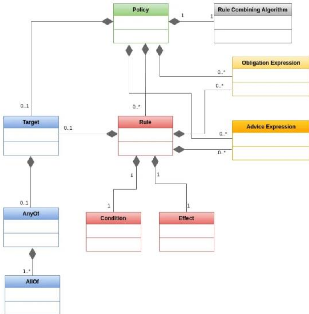
Εικόνα 2.3 Αρχιτεκτονική XACML[13]
