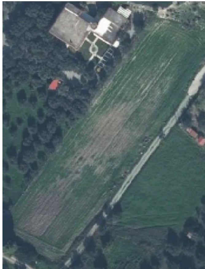
Εικόνα 5. Δορυφορική Απεικόνιση του αγροτεμαχίου στην περιοχή Ροβιές
