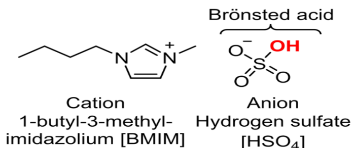
Εικόνα 60: Μοριακή δομή του όξινου θειικού 1-βουτυλ-3-μεθυλιμιδαζόλιου (Raubert, et al., 2019)
