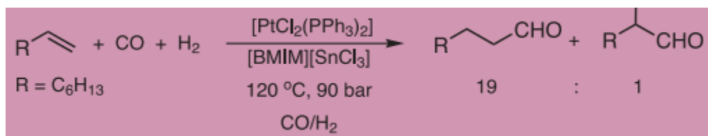
Εικόνα 26: Υδροφορμυλίωση (Δούκα, 2012)
