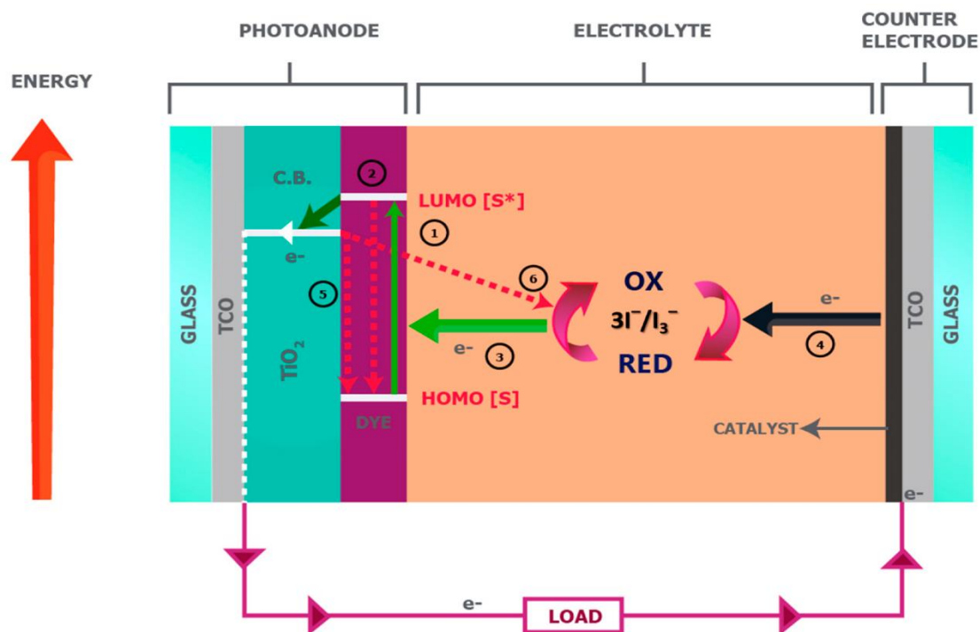
Εικόνα 45: Μηχανισμός λειτουργίας ενός τυπικού ηλιακού κυττάρου ευαισθητοποιημένου με βαφή (Iftikhar, Sonai, Hashmi, Nogueira, & Lund, 2019)
