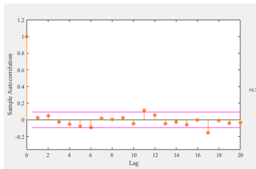
Εικόνα 56: HLT Autocorrelation,
