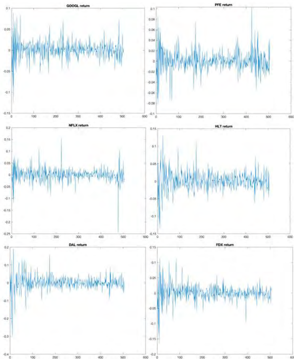
Εικόνα 16: Stocks log
