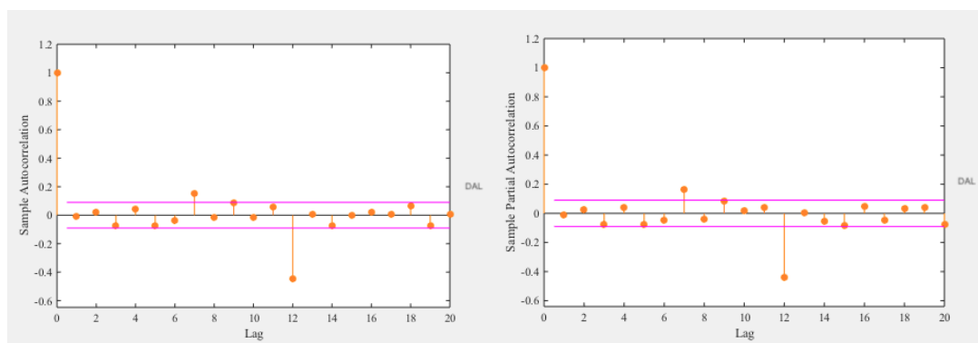
Εικόνα 62: DAL Autocorrelation,
