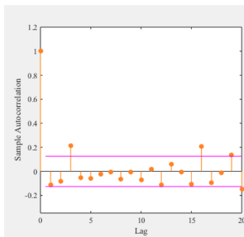
Εικόνα 41: PFE Autocorrelation,
