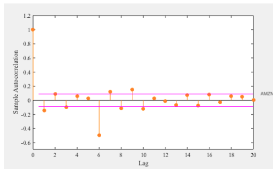
Εικόνα 27: AMZN Autocorrelation,
