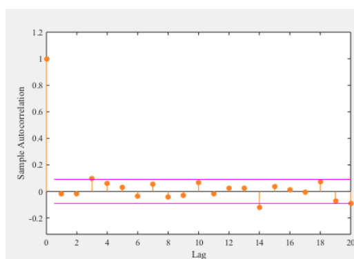
Εικόνα 76: TSLA Autocorrelation,
