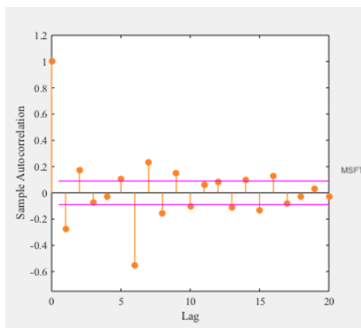
Εικόνα 31: MSFT Autocorrelation,
