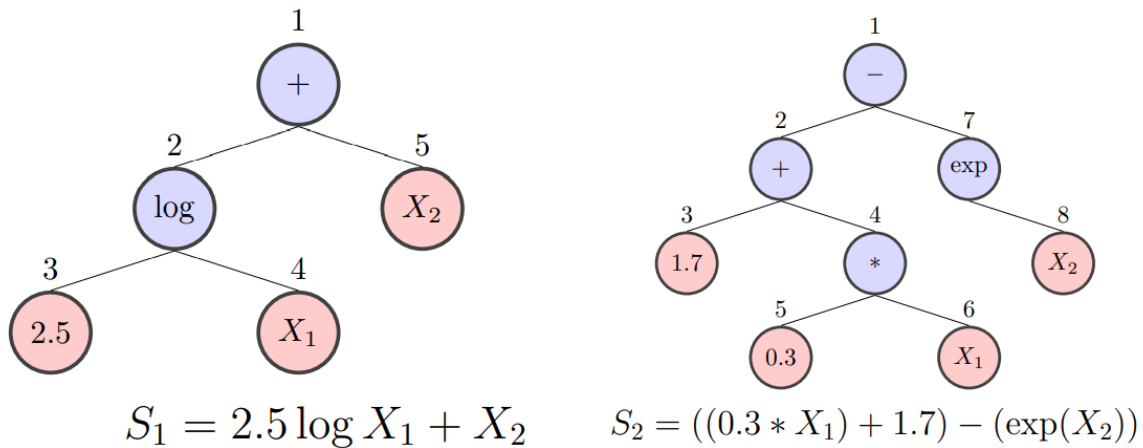
Σχήμα 17: Παραδείγματα συμβολικών εκφράσεων S_1 και S_2 .
