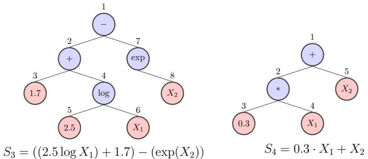
Σχήμα 18: Παραδείγματα συμβολικών εκφράσεων S_3 και S_4 .
