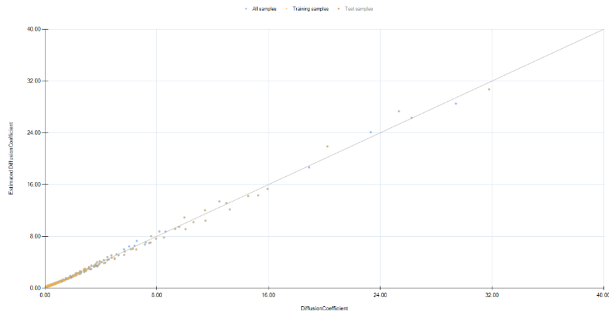
Σχήμα 24: Γράφημα ταυτότητας (identity plot) της Εξ. F_8 του Πίνακα 8.
