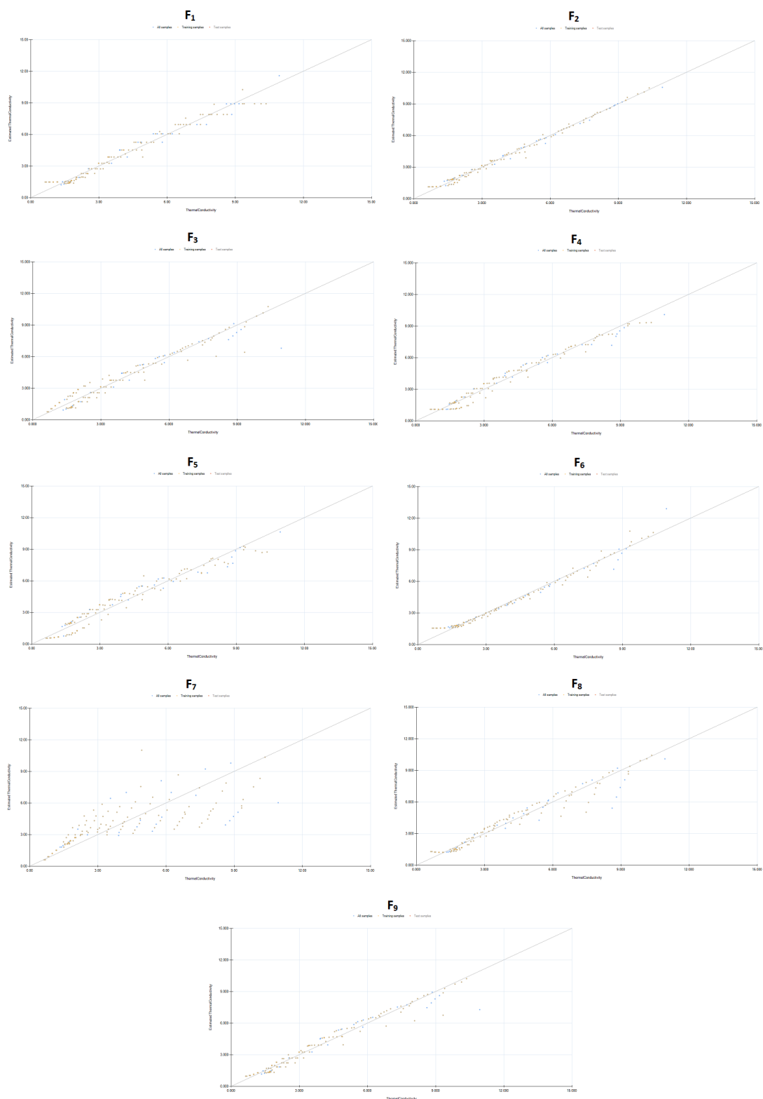
Σχήμα 32: Γραφήματα διασποράς για τις εξισώσεις F_i ( i = 1, \dots, 9 ) του Πίνακα 12 (θερμική αγωγιμότητα \lambda ).
