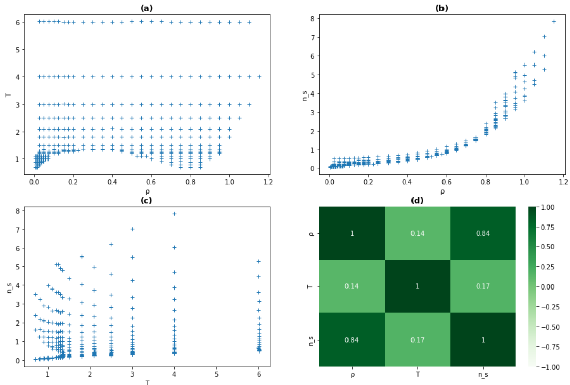
Σχήμα 25: Συμπεριφορά των δεδομένων. (α) Διάγραμμα φάσης \rho - T . (β) Διάγραμμα \rho - n_s . (γ) Διάγραμμα T - n_s . (δ) Τιμές συντελεστή συσχέτισης για τις μεταβλητές \rho, T, n_s .
