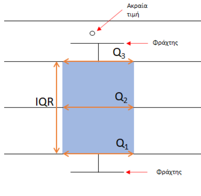
Σχήμα 5: Μορφή Θηκογράμματος (box-plot).
