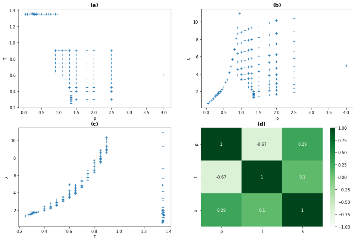
Σχήμα 28: Συμπεριφορά των δεδομένων. (a) Διάγραμμα φάσης \rho - T . (b) Διάγραμμα \rho - \lambda . (c) Διάγραμμα T - \lambda . (d) Τιμές συντελεστή συσχέτισης για τις μεταβλητές \rho, T, \lambda .
