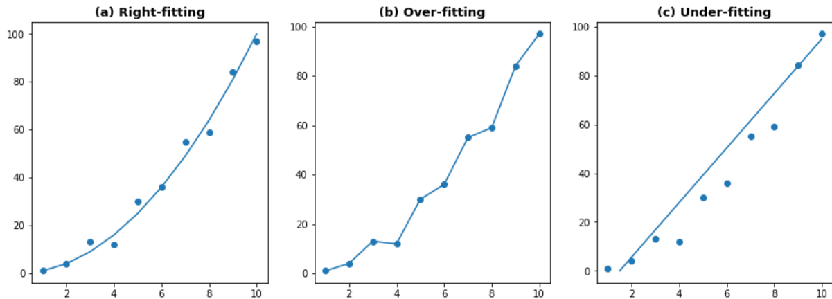
Σχήμα 4: Παράδειγμα ταιριάσματος μοντέλων στα δεδομένα. α) Κανονική προσαρμογή του μοντέλου σε ένα τυχαίο σετ δεδομένων. β) Υπερπροσαρμογή του μοντέλου στα δεδομένα. γ) Υποπροσαρμογή του μοντέλου στα δεδομένα.
