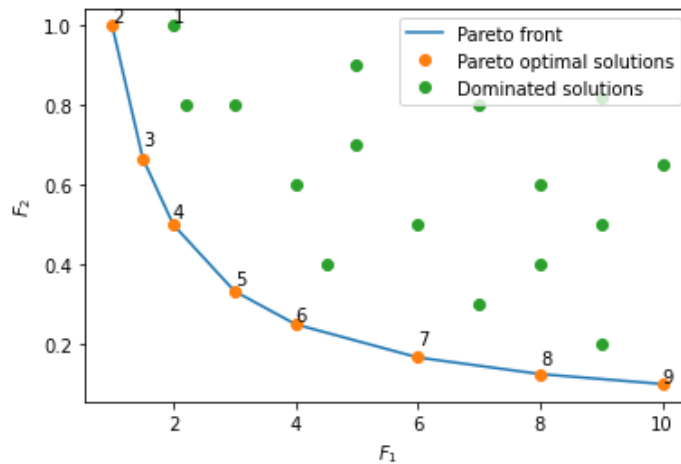
Σχήμα 20: Παράδειγμα Pareto front.
