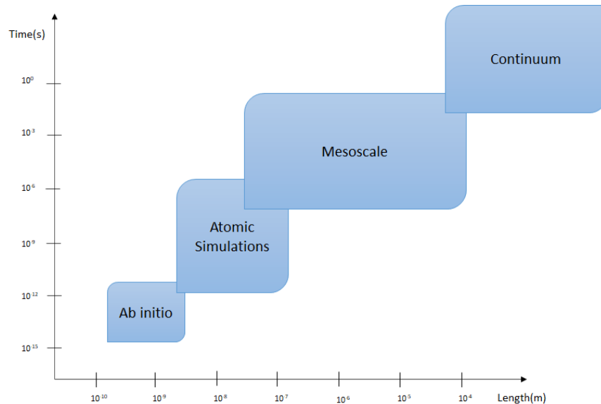
Σχήμα 21: Πολλαπλή κλίμακα της Επιστήμης των Υλικών και μέθοδοι που χρησιμοποιούνται.
