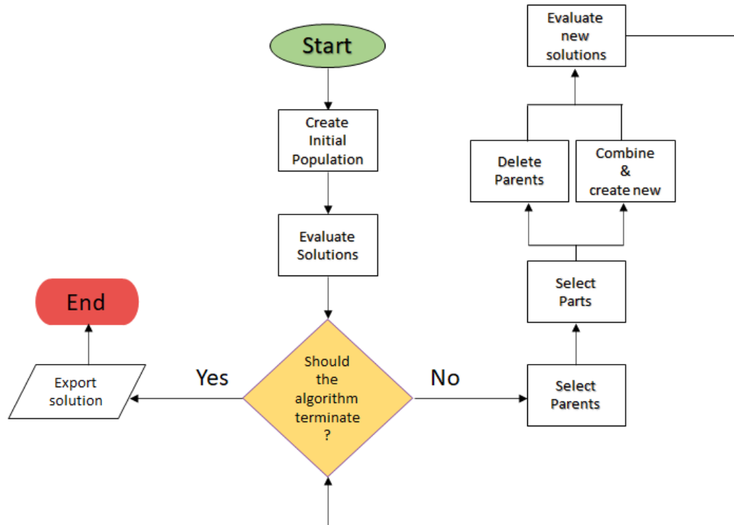
Σχήμα 19: Διαδικασία συμβολικής παλινδρόμησης μέσω γενετικού προγραμματισμού.
