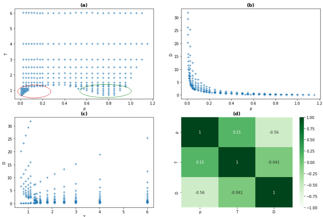
Σχήμα 23: Συμπεριφορά των δεδομένων συντελεστή διάχυσης D . (α) Διάγραμμα φάσης \rho - T . Η κόκκινη περιοχή απεικονίζει την αέρια κατάσταση (gas), η πράσινη περιοχή την υγρή (liquid) ενώ όλη η άλλη περιοχή είναι η υπερκρίσιμη (super critical). (β) Διάγραμμα \rho - D . (γ) Διάγραμμα T - D . (δ) Τιμές συντελεστή συσχέτισης για τις μεταβλητές \rho, T, D .
