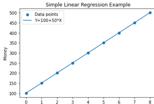
Σχήμα 8: Παράδειγμα ταιριάσματος (fitting) της εξίσωσης απλής γραμμικής παλινδρόμησης Y = 100 + 50 * X στο σετ δεδομένων του Πίνακα 2.
