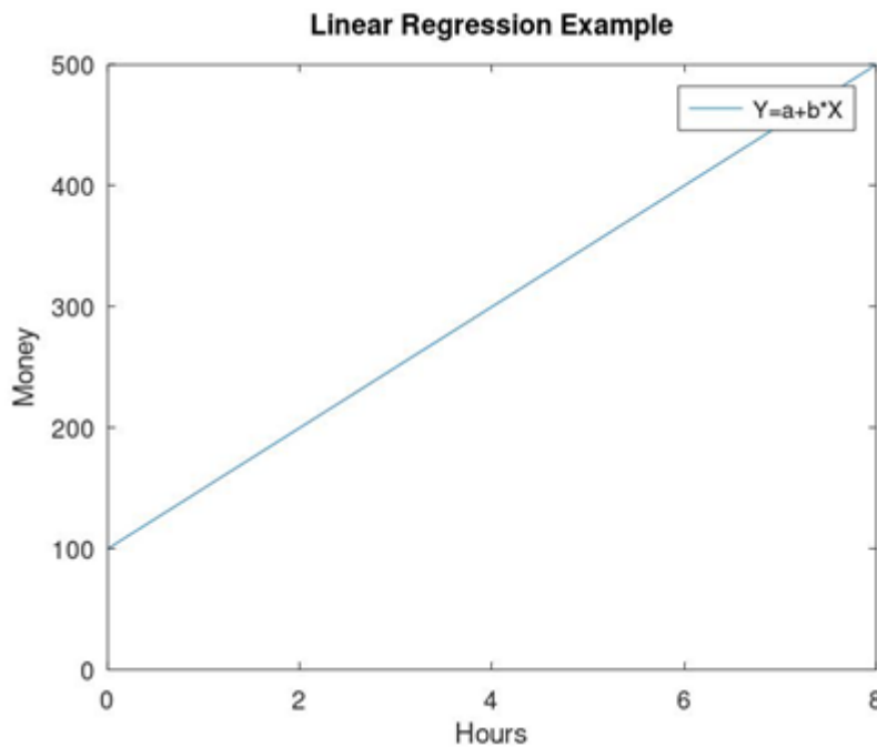
Σχήμα 6: Παράδειγμα γραμμικής παλινδρόμησης. Ο άξονας των Χ αποτυπώνει την κάθε ώρα, όπου 0 είναι η αρχική μέτρηση στις 12:00 και 8 είναι η τελική μέτρηση στις 20:00. Ο άξονας των Y αποτυπώνει τον αριθμό των χρημάτων που υπάρχουν στο ταμείο.
