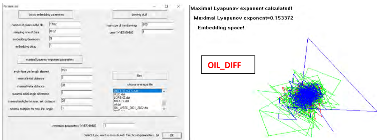
Γράφημα 5.17. Μέγιστος εκθέτης πρώτων διαφορών. Πηγή: Ιδία επεξεργασία (lyarpmx.exe).
