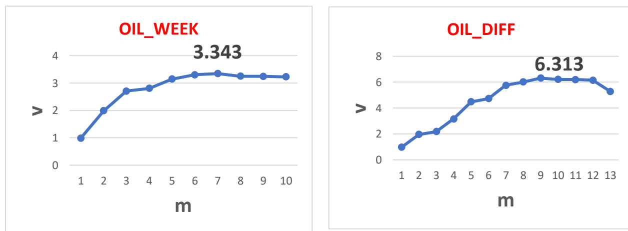
Γράφημα 5.7. Διάσταση συσχέτισης v και εμβύθισης m με τη μέθοδο των Grassberger -Procaccia (1983). Πηγή: Ιδία επεξεργασία (Fractan, Excel).
