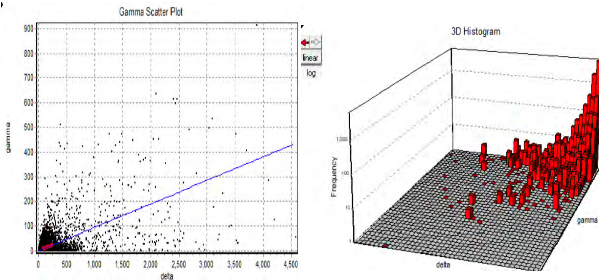
Γράφημα 6.2. Διάγραμμα διασποράς και τρισδιάστατο ιστόγραμμα κατανομής του θορύβου.
