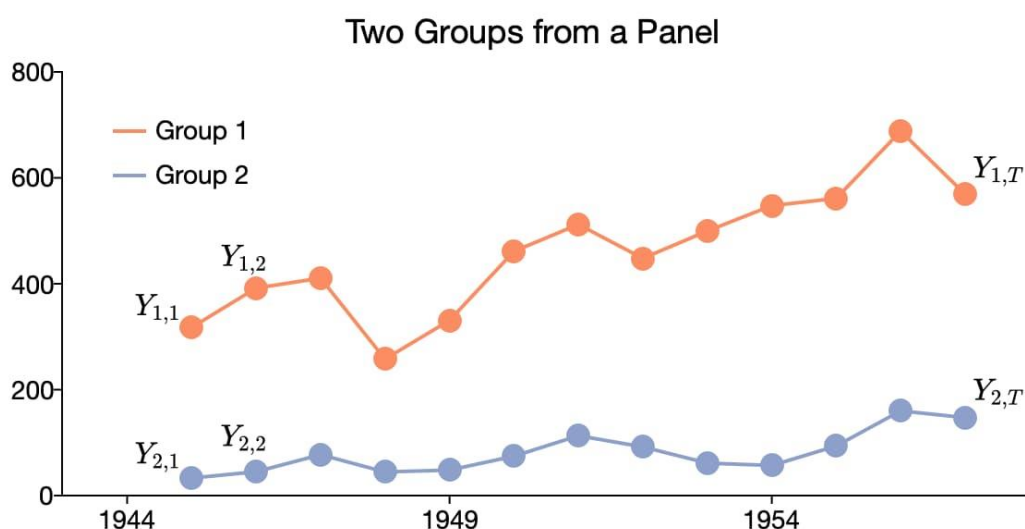
Σχήμα 92: Ομάδες δεδομένων panel
