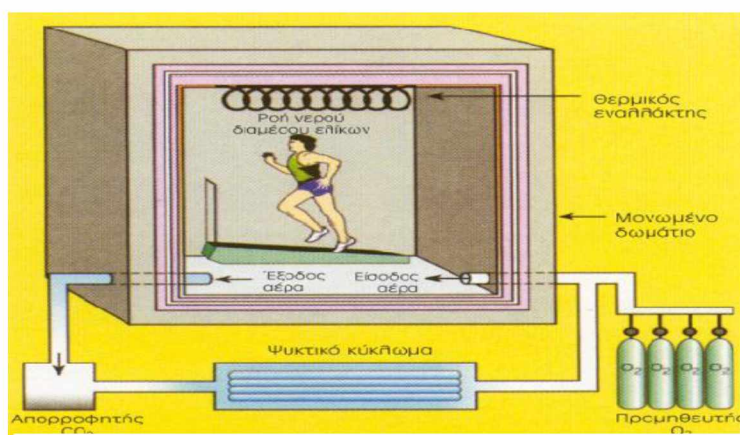
Εικόνα 2.1 Άμεση θερμιδομετρία
