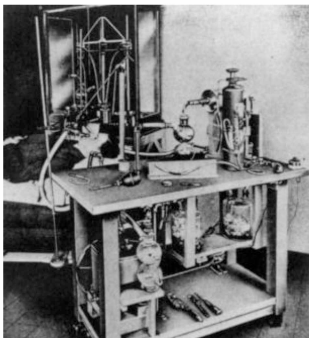
Εικόνα 2.2 Έμμεσο θερμιδόμετρο
