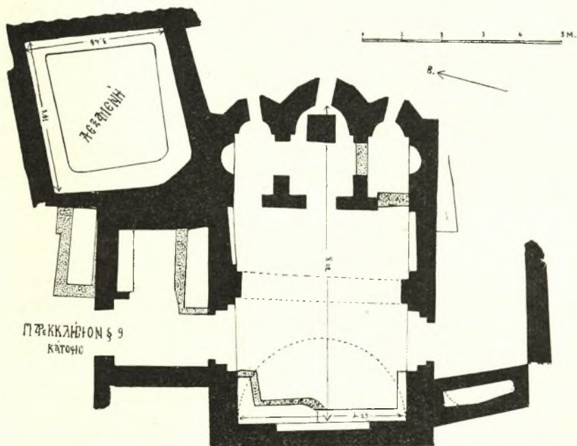
Εἰκ. 13. Κάτοψις τοῦ ναοῦ § 9 τῶν «Ταξιάρχων».
