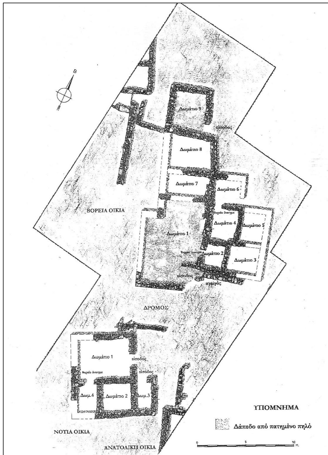
Εικ. 16: Διμήνη, Τομέας II: Κάτοψη μυκηναϊκών αρχιτεκτονικών καταλοίπων της Βόρειας, Νότιας και Ανατολικής Οικίας.
