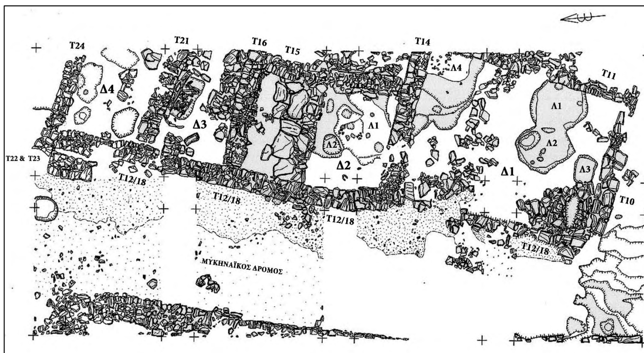
Εικ. 57: Κάτοψη μυκηναϊκών αρχιτεκτονικών καταλοίπων στη θέση Μακρυχώρι (Λάρισα): Βόρειο κτίριο (Περίοδος V:ΥΕ ΙΙΒ2/ΥΕ ΙΙΙΓ).
