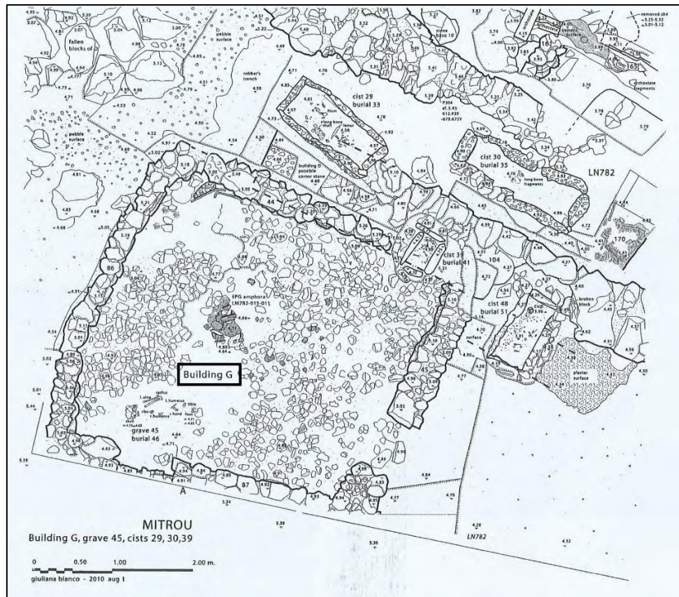
Εικ. 28: Κάτοψη μυκηναϊκών αρχιτεκτονικών καταλοίπων του οικισμού στη θέση Μήτηρου (Φθιώτιδα): Κτίριο G.
