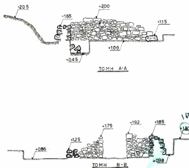
Εικ. 10 Σχεδιαστική αποτύπωση των τόμων της ανασκαφής με τα βάθη τους.
