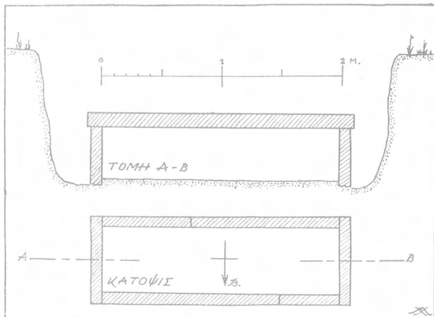
Εἰκ. 9. Σχέδιον κατόψεως καὶ τομῆς τάφου, εὐρεθέντος παρὰ τὴν Τοῦμπαν (Θεσσαλονίκη)
