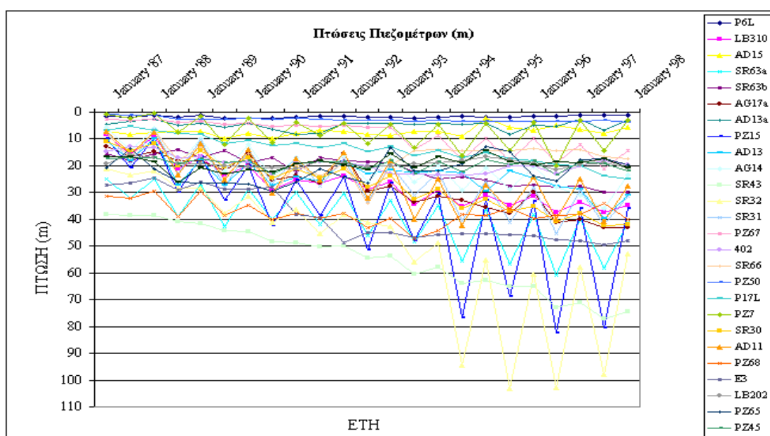
Σχήμα: 1.3 Διαγράμματα πτώσης στάθμης πιεζομέτρων 87-97
