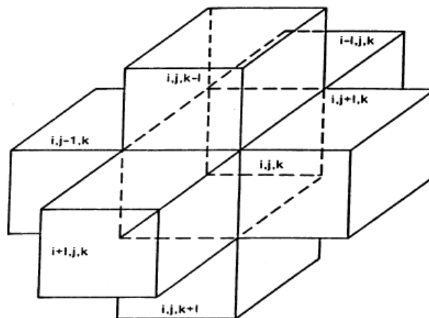
Σχήμα 3.3: Το κελί (i,j,k) και τα γειτονικά του.
