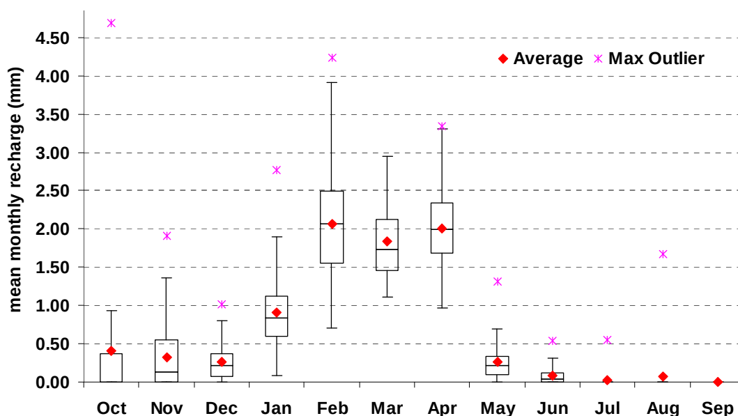
Σχήμα 4.18:Θηκόγραμμα μηνιαίας κατείσδυσης για την περίοδο 2009 έως 2058 για το σενάριο A2.
