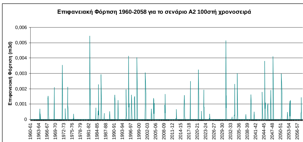
Σχήμα 4.16: Η100στή χρονοσειρά κατεισδυσης, περίοδος 1960-2058
