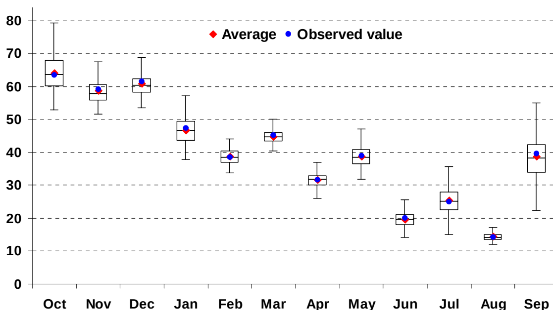
Σχήμα 4.5: Θηκόγραμμα καταβιβασμένης βροχόπτωσης για την ιστορική περίοδο.
