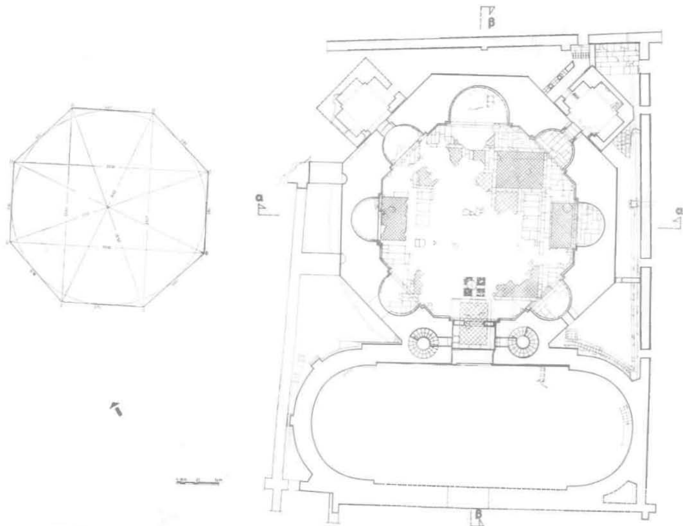
Σχ. 10. 'Οκτάγωνο. 'Υπάρχουσα κατάσταση, κάτωψη. 'Αριστερά, οί κύριες διαστάσεις της οκταγωνικής αίθουσας.
