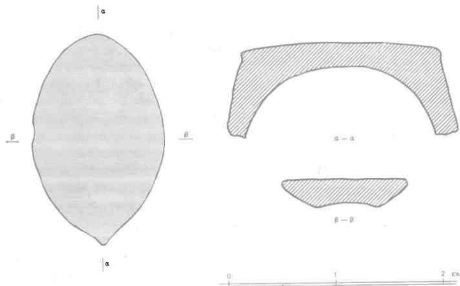
Σχ. 1. Κάτοψη και τομές της σφενδόνης του δαχτυλιδιού M 842.
