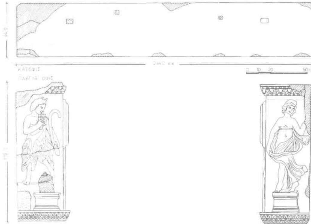
Σχ. 2. Άνασκαφή οικοπέδου οδού Ίσαύρων. Νότια στοά. Μαρμάρινο διακοσμητικό τόξο.
