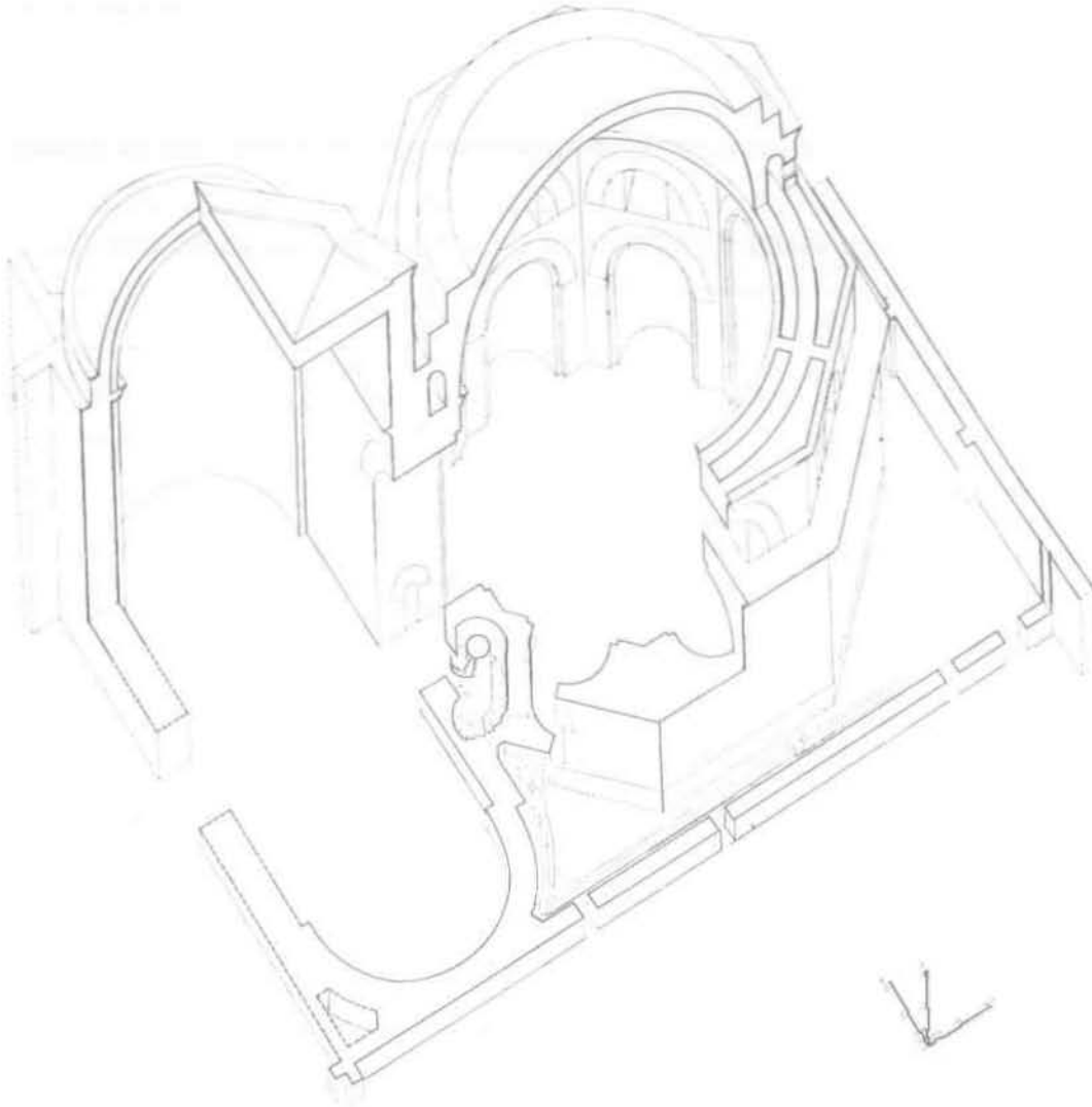
Σχ. 20. Τό όκτάγωνο στήν ύστερορωμαϊκή φάση. Γραφική αποκατάσταση τοῦ συνόλου (α' λύση). Ἐξονομετρικό.
