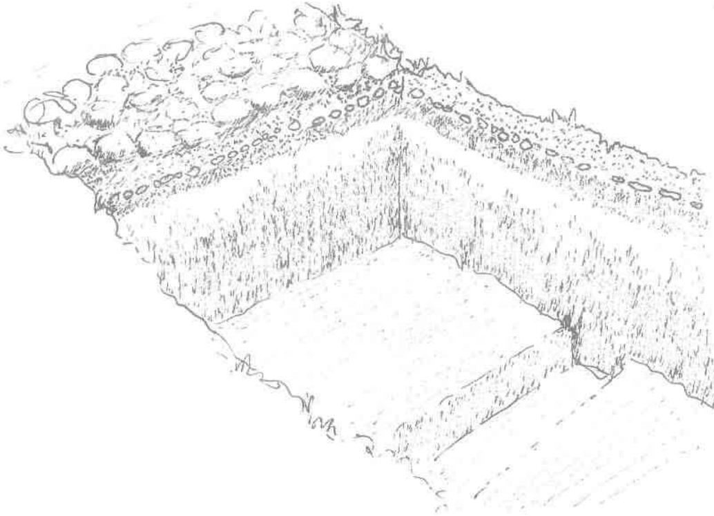
Σχ. 10. Μωσαϊκὸ δάπεδο τῆς Ἀμαζονομαχίας. Στρωματογραφία (σχέδιο τοῦ συγγραφέα).
