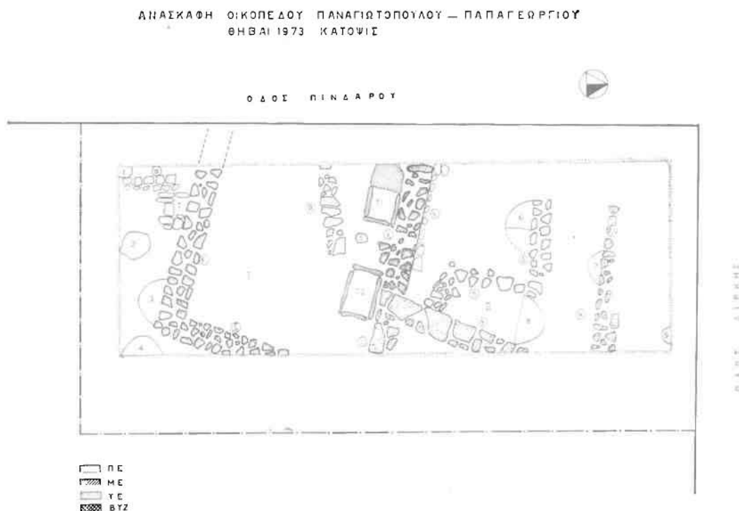
Σχ. 2. Κάτοψη της άνασκαφής του οικοπέδου Παναγιωτοπούλου-Παπαγεωργίου, Θήβα 1973.
