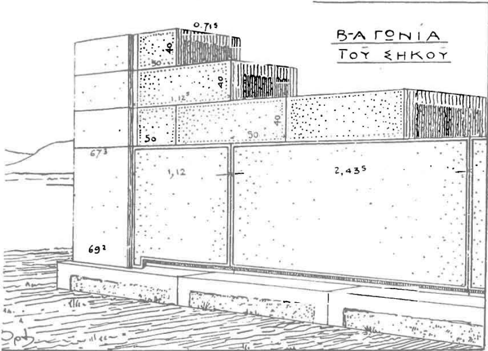
Εἰκ. 22. Παραστάς, ὀρθοστάται καὶ πλίνθοι τοῦ σηκοῦ (ΒΑ γωνία).
