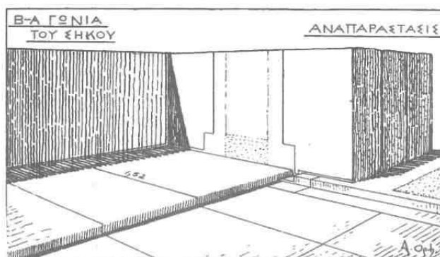
Εἰκ. 32. Ἀναπαράστασις τῆς ΒΑ. γωνίας τοῦ σηκοῦ (ἄνευ κιόνων καὶ παραστάδων).
