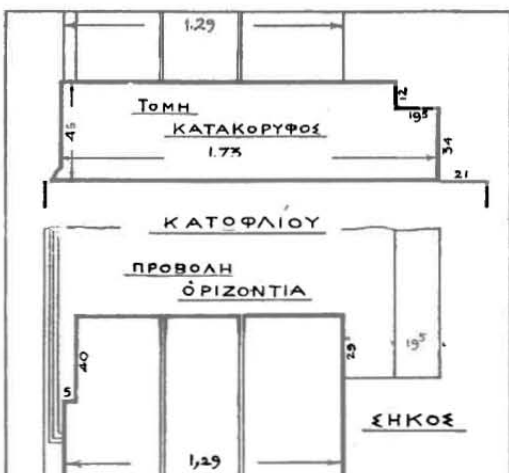
Εἰκ. 28. Λεπτομέρεια τοῦ οὐδοῦ καὶ τοῦ σηκοπροδ. τοίχου.
