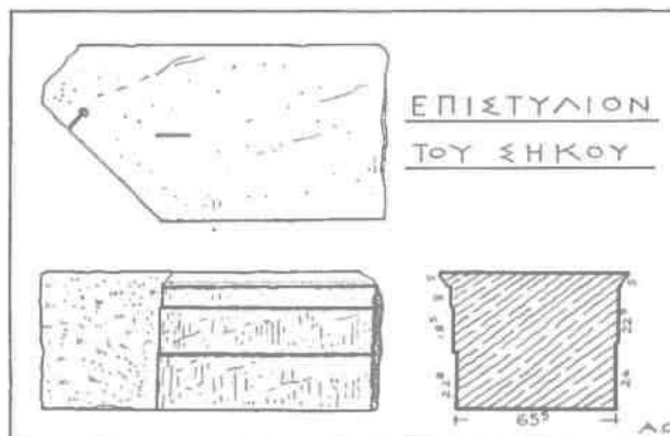
Εἰκ. 34. Ἐπιστύλιον τοῦ σηκοῦ.
