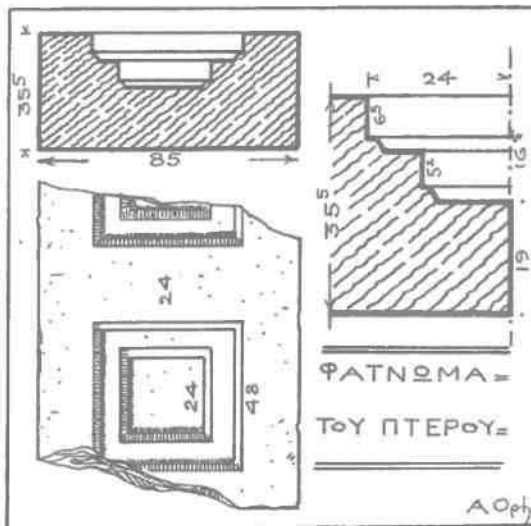
Εἰκ. 26. Φάτνωμα τοῦ πτεροῦ
