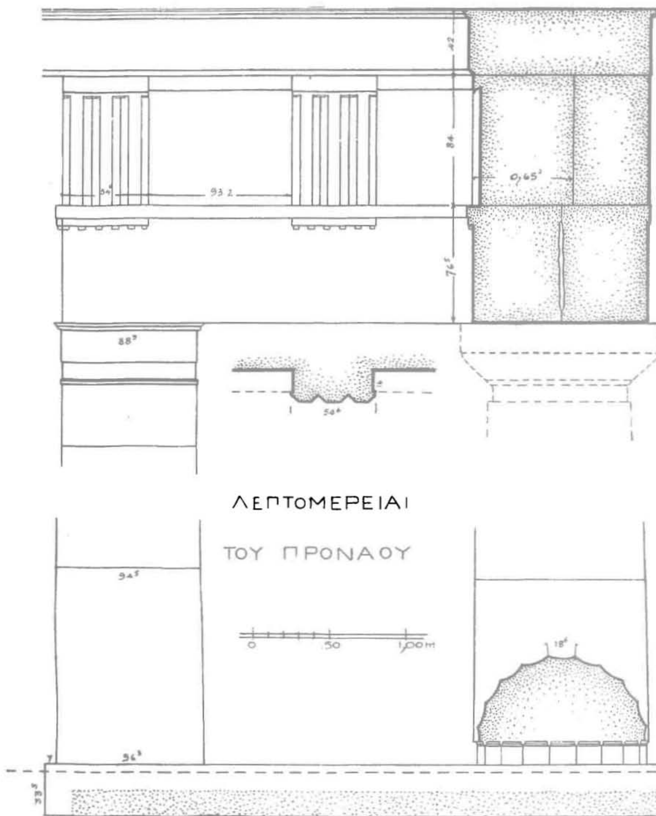
Εἰκ. 17. Στοιχεῖα τῆς προσόψεως τοῦ προναοῦ.
