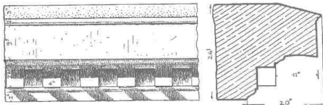
Εἰκ. 36. Γεῖσον τοῦ σηκοῦ. Πρόσοψις καὶ τομῆ.
