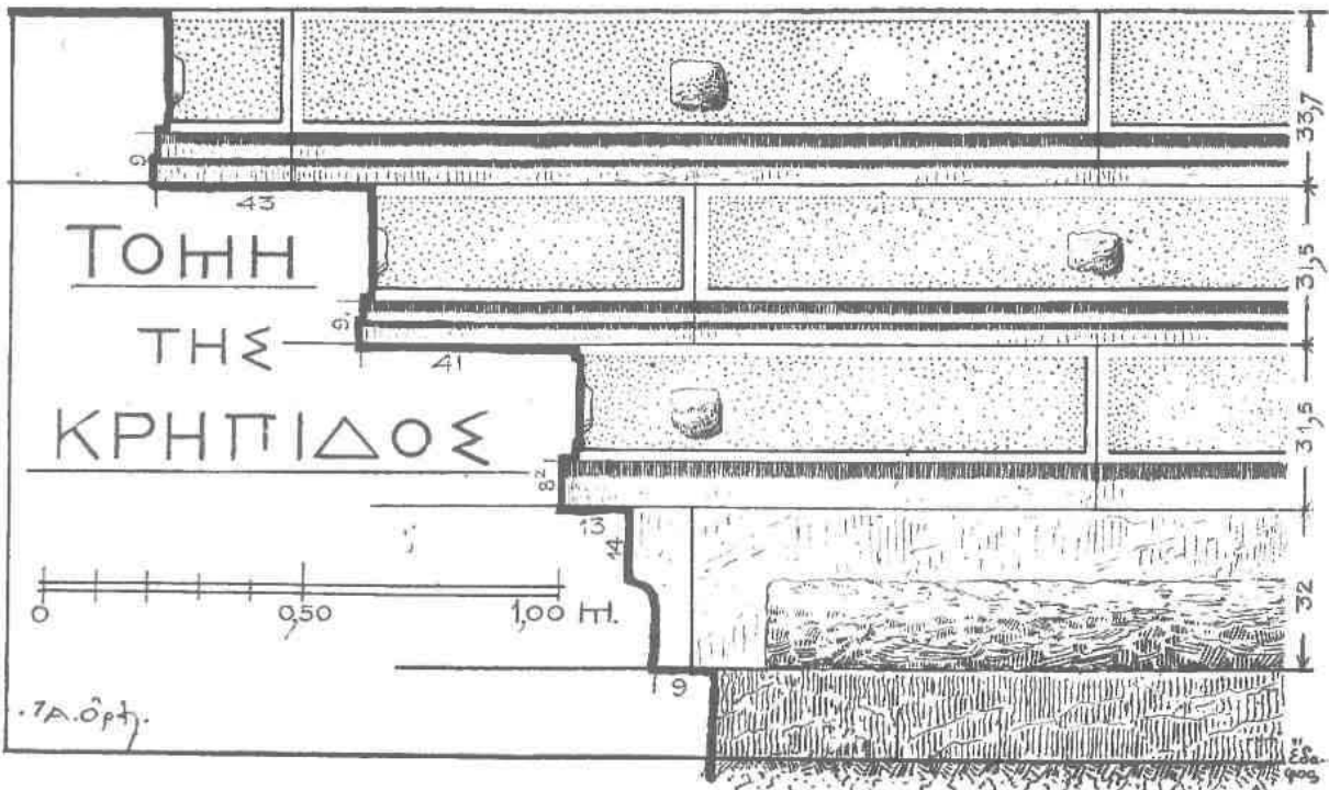
Εἰκ. 3. Λεπτομέρεια καὶ τομὴ τῆς κρηπίδος.
