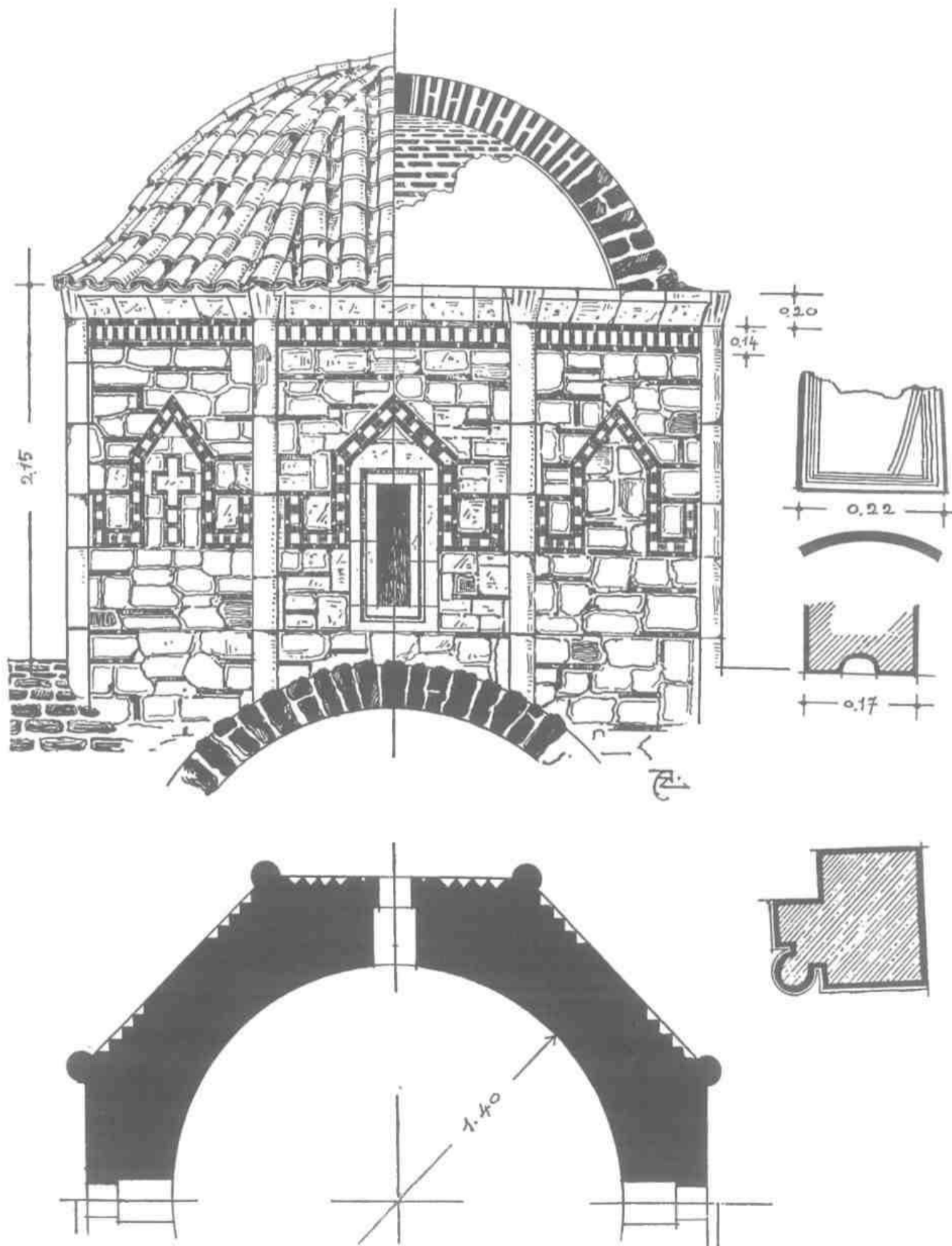
Είκ. 3. Τοιχοδομία ναού παλαιᾶς Μονῆς Φιλοσόφου.
