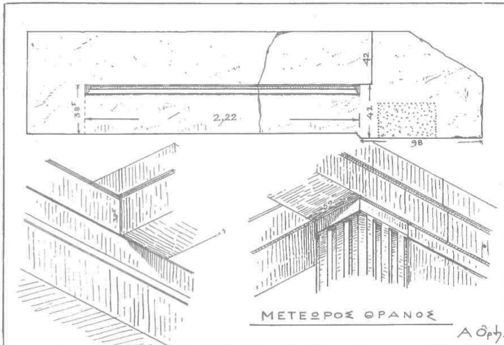
Εἰκ. 21. Μετέωρος θράνος.
