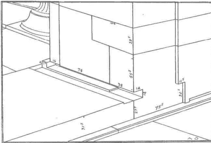
Εἰκ. 40. Λεπτομέρεια τοῦ σταθμοῦ τῆς θύρας τοῦ ἐν Φιγαλεΐᾳ ναοῦ.
