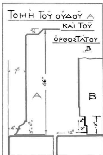
Εἰκ. 27. Τομή τοῦ οὐδοῦ καὶ τῶν ὀρθοστατῶν τοῦ προδῶμου.
