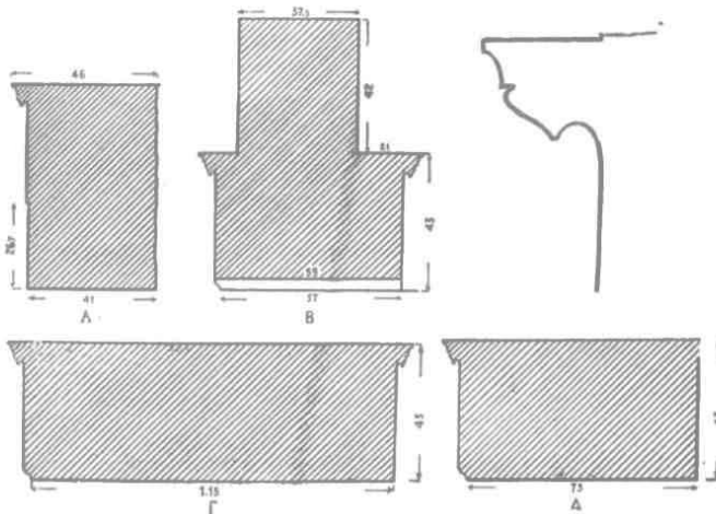
Εἰκ. 20. Τομαὶ τῶν θράνων.
