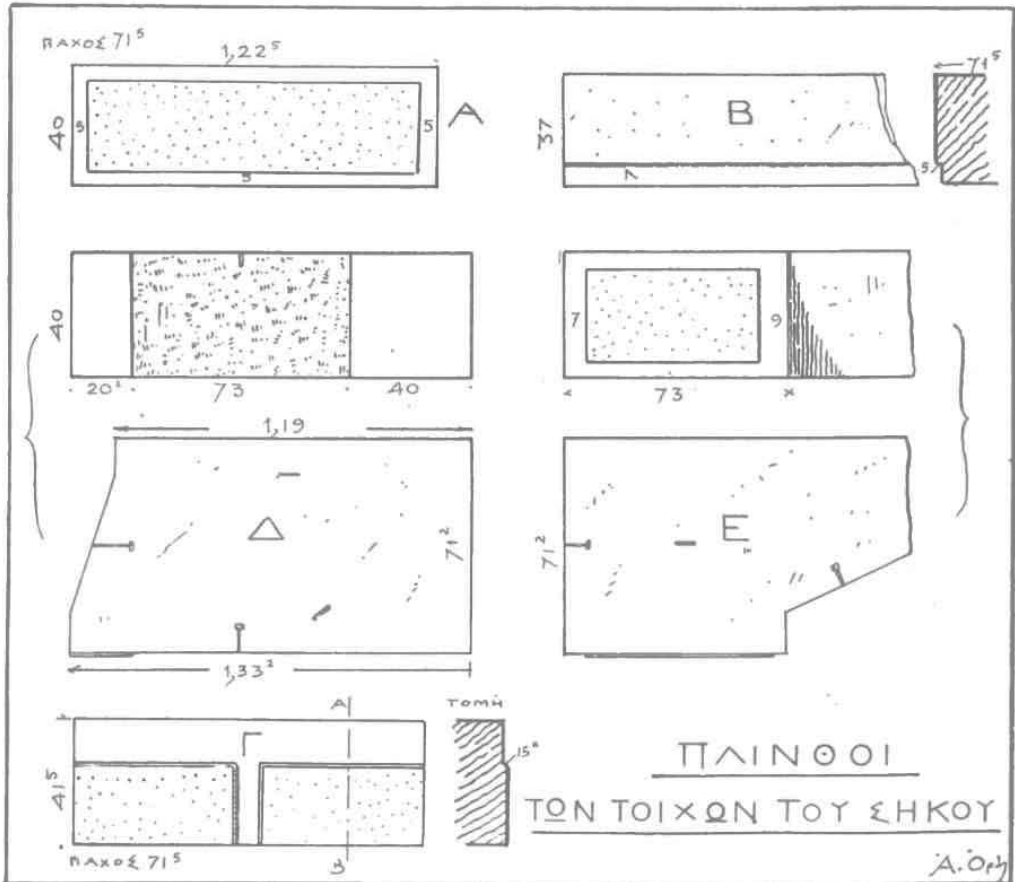
Εἰκ. 25. Πλίνθοι τῶν τοίχων τοῦ σηκοῦ.
