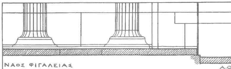
Εἰκ. 41. Τομή κατὰ τὸν ἄξονα τοῦ σηκοῦ.
