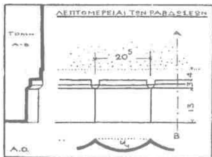
Εἰκ. 4. Δεπτομέρεια ραβδώσεως τῶν κατωτάτων σφονδύλων.
