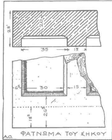
Εἰκ. 37. Φάτνωμα ἐκ τῆς ὀροφῆς τοῦ σηκοῦ.
