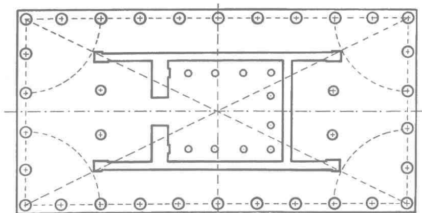
Εἰκ. 42. Γραφικὴ κατασκευὴ τῆς κατόψεως τοῦ ἐν Στράτῳ ναοῦ.
