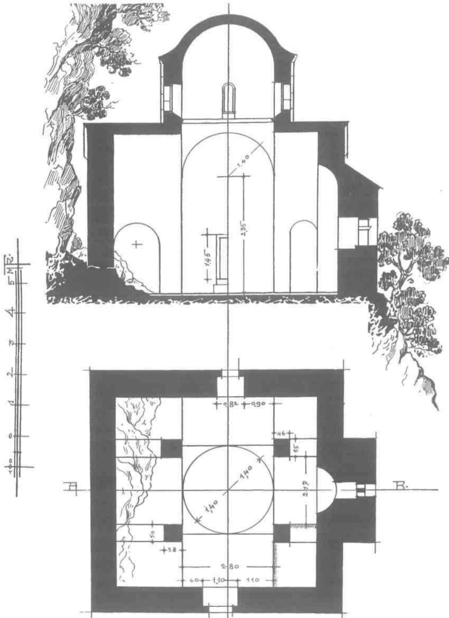
Εικ. 2. Κάτοψις και τομή παλαιᾶς Μονῆς Φιλοσόφου.
