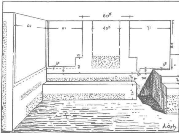
Εἰκ. 31. Ἡ ΒΑ γωνία τοῦ σηκοπροδομίου τοίχου.
