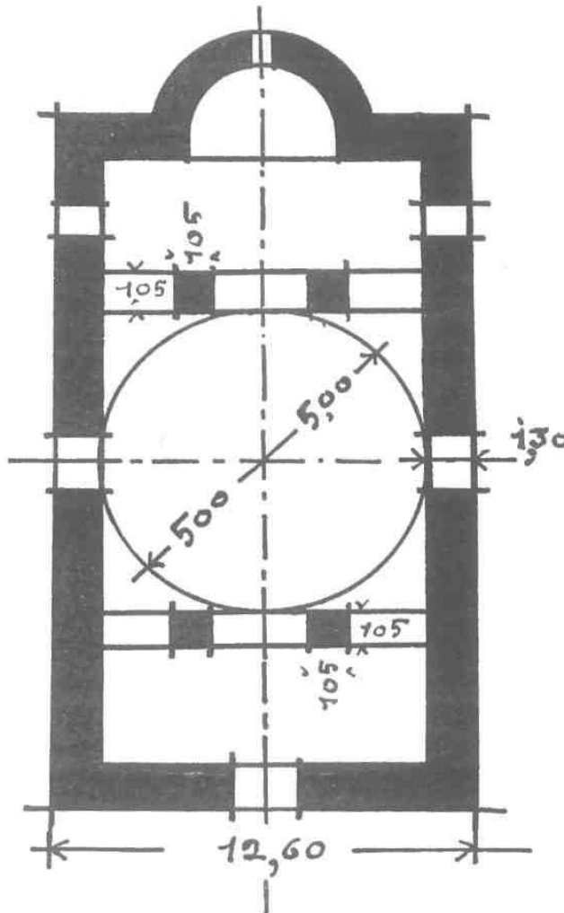
Εἰκ. 7. Κάτοπις ναοῦ Ἁγίας Κυριακῆς Δημητσάνης.
