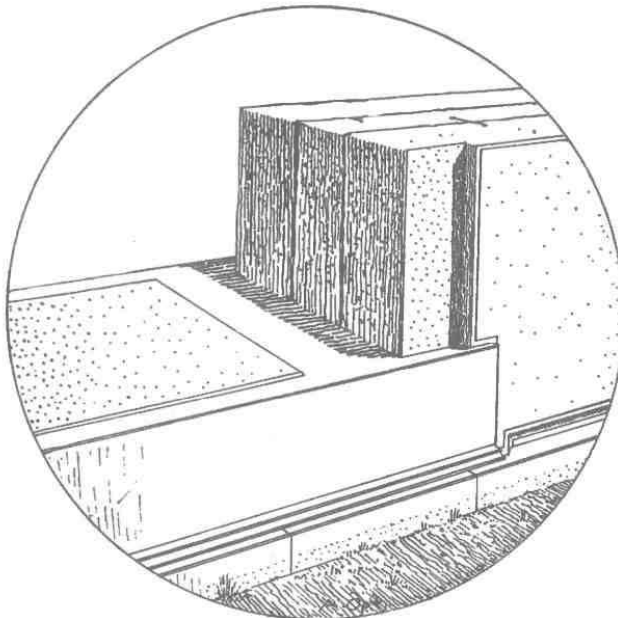
Εἰκ. 29. Τμήμα τοῦ οὐδοῦ μετὰ τῶν σηκοπροδομίων ὀρθοστατῶν.
