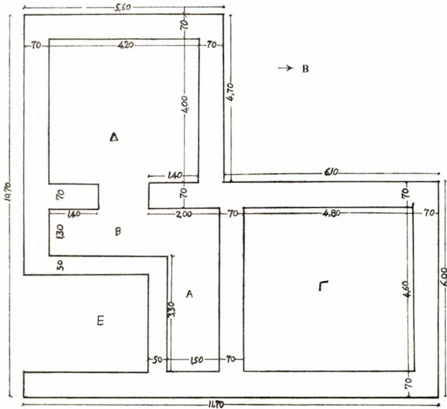
Σχ. 1. Κάτωις Ρωμαϊκῆς ἐπαύλεως, ἀποκαλυφθείσης εἰς οἰκόπεδον Παρασκευοπούλου εἰς Σπάρτην
