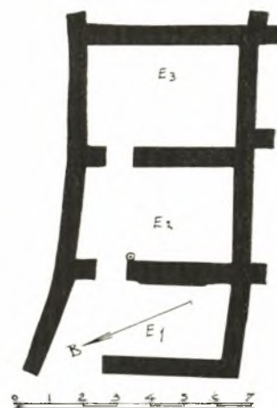
Εἰκ. 3. Οἶκημα Ε (Σχέδιον τοῦ Τραυλοῦ).
