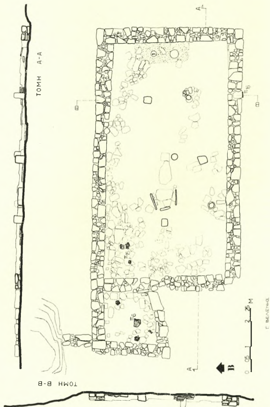
Σχέδ. 8. Νάξος. Τσικαλαριό. Ὁρθογώνιον κτήριο
