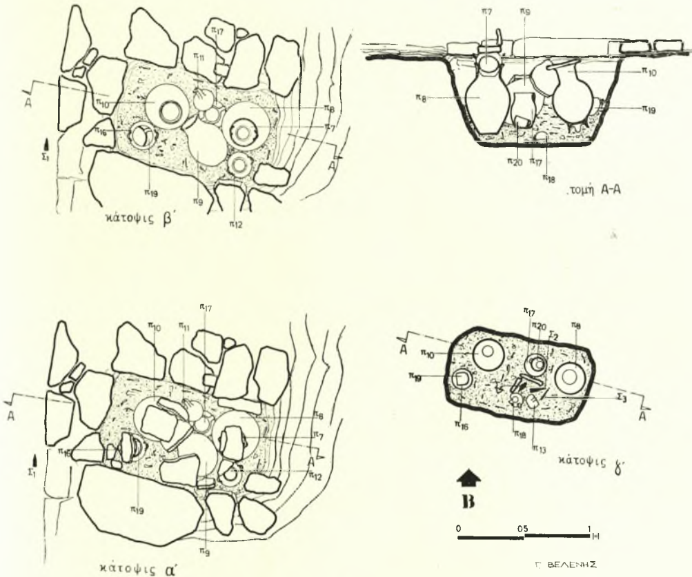
Σχέδ. 6. Τάφος τύμβου 14 εἰς Τσικαλαριό Νάξου
