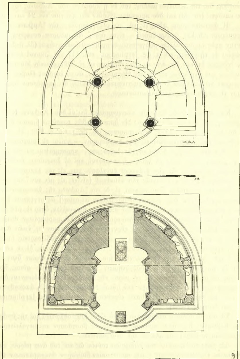
Εἰκ. 1-2. Κάτοψις βάσεως καὶ ἄνω δαπέδου τοῦ Ἄμβωνος τῆς Θεσσαλονίκης.
