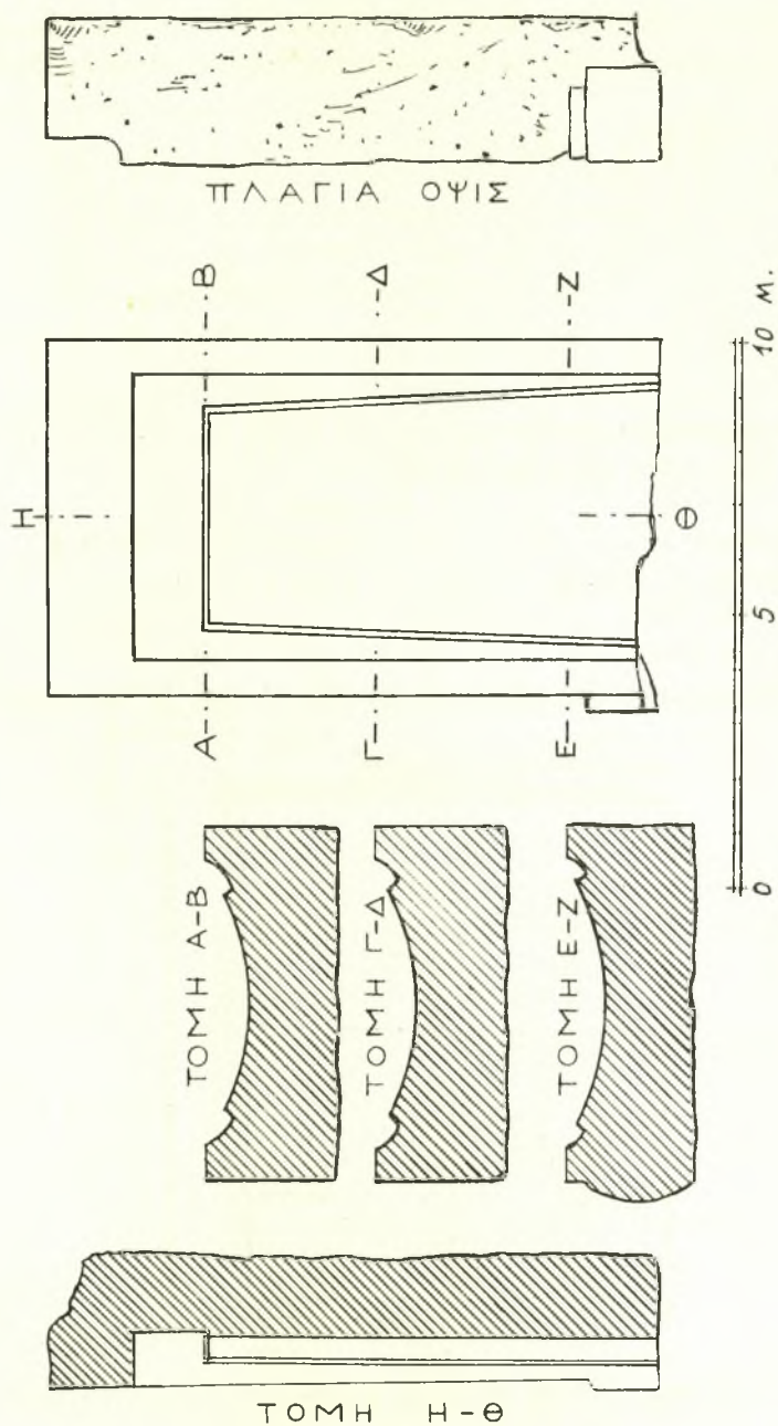
Fig. 8. Τομαί, πρόσφυς καὶ πλαγία ὄψις τοῦ παραδειγματος τῶν κεράμων.
