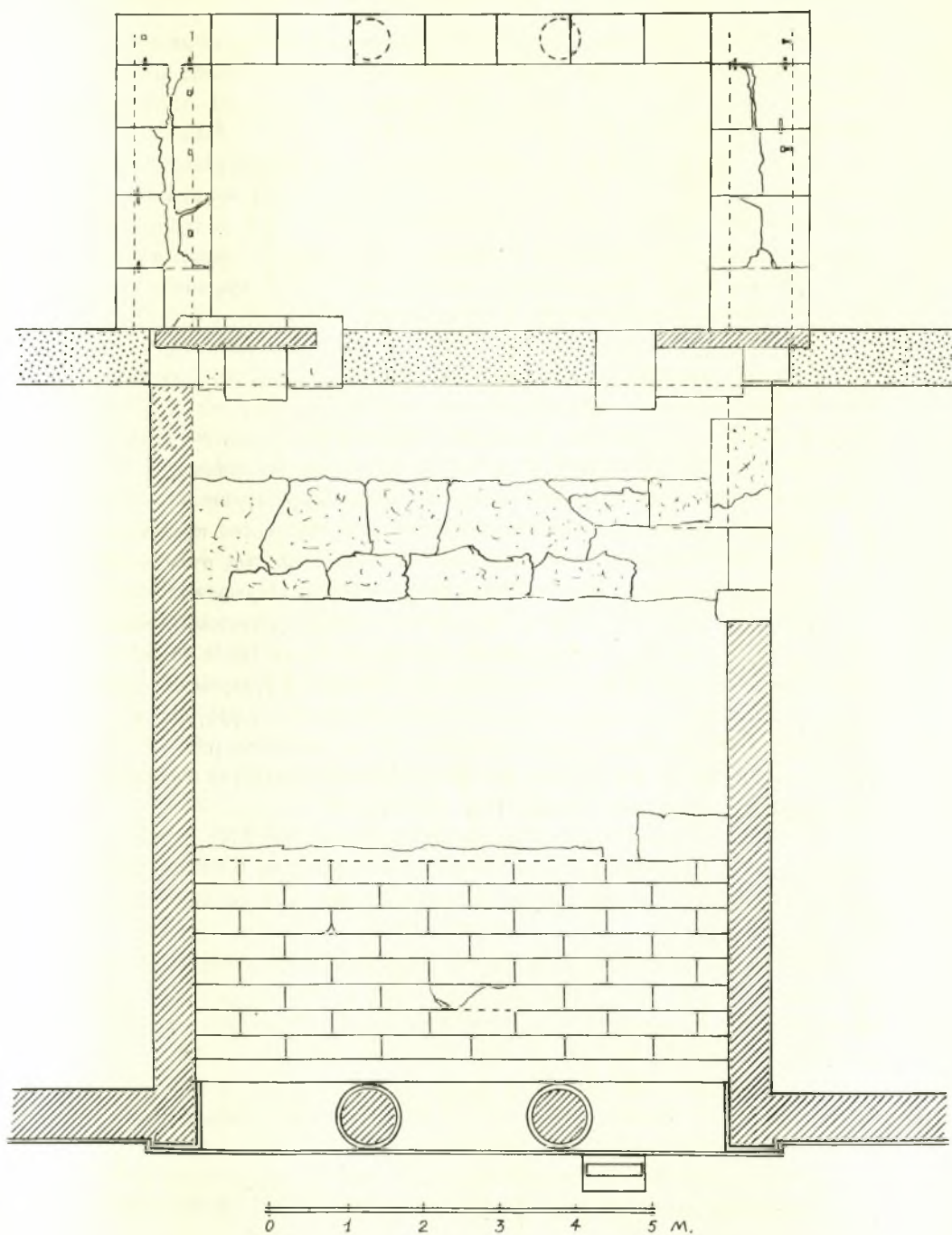
Εικ. 5. Κάτοψις τῆς μνημειώδους κλίμακος εισόδου μετὰ τὸν ὀλοσχερῇ καθαρισμὸν τῆς.
