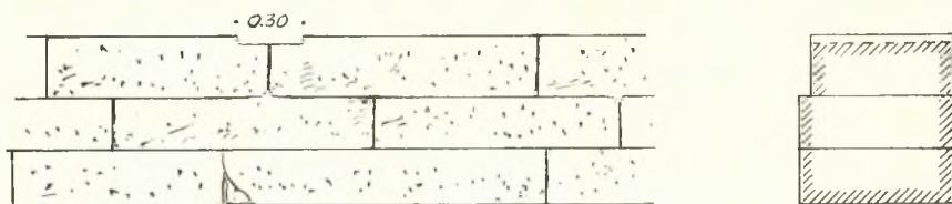
Εἰκ. 2. Τὸ ἄνω μέρος τοῦ ὀπισθίου τοίχου τοῦ οἴκου. Ὅψις καὶ τομή.
