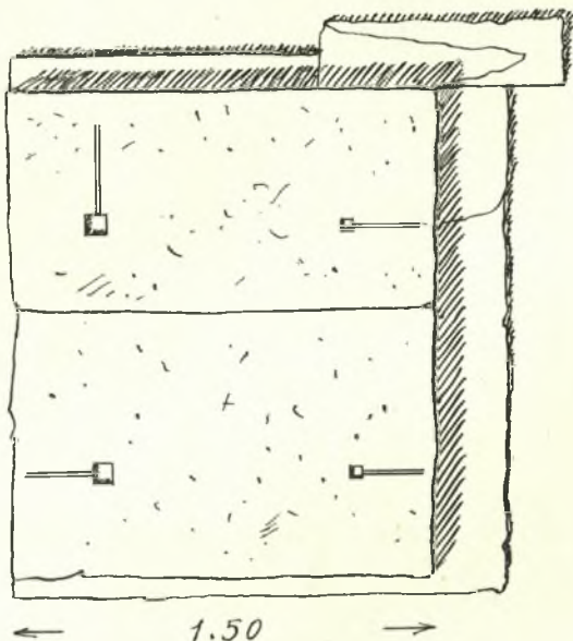
Εἰκ. 10. Κάτοψις τοῦ ἐν τῷ κέντρῳ τῆς περιστύλου αὐλῆς εὐρεθέντος θεμελίου.
