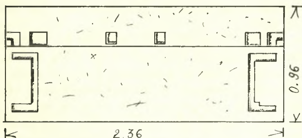
Εἰκ. 6. Κάτοψις τοῦ κεντρικοῦ κατωφλίου τῶν μετακινίων τῆς κλίμακος.
