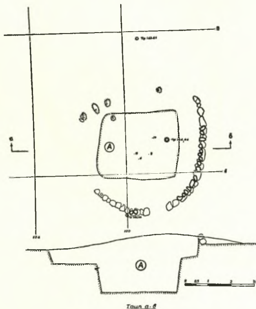
Σχεδ. 34. Ὁ τύμβος XXVIII
