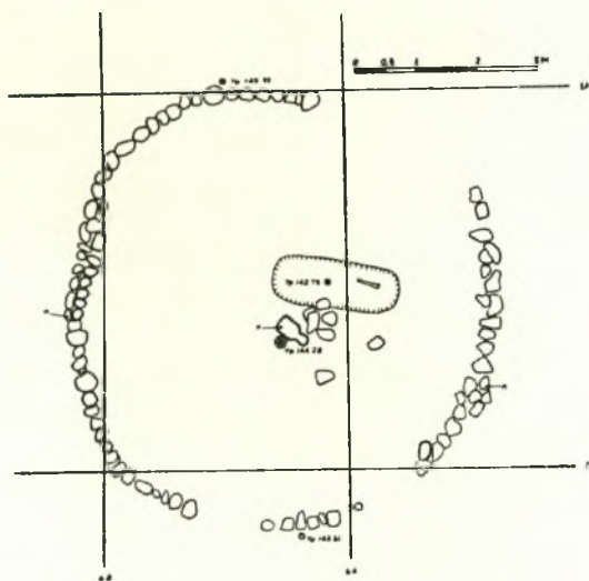
Σχεδ. 25. Ὁ τύμβος XIX
