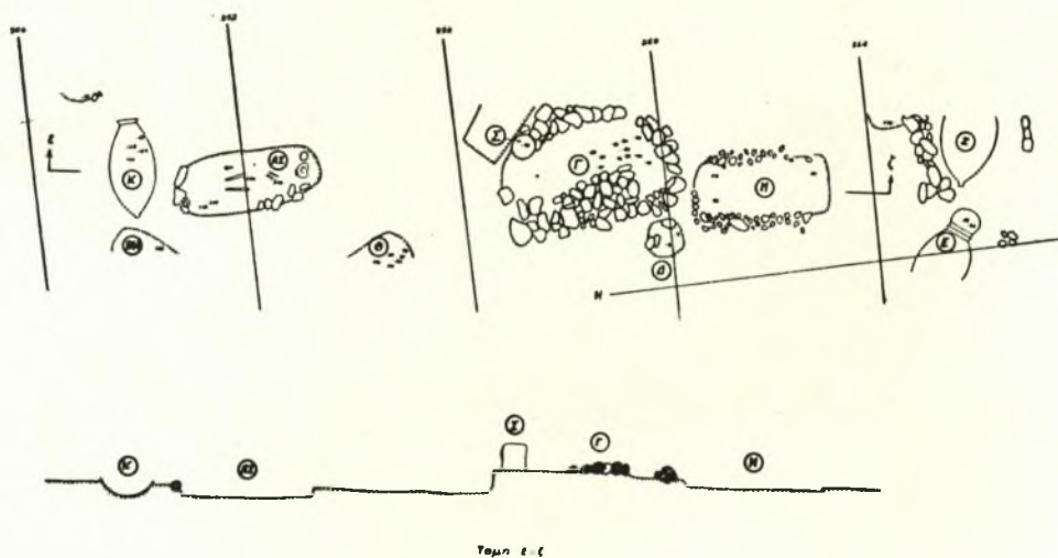
Σχεδ. 50. Τομή ε-ζ τοῦ τύμβου LXV
