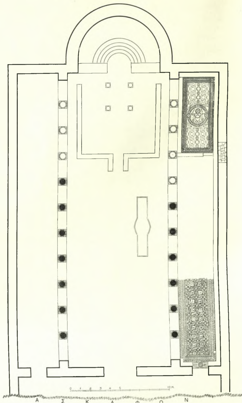
Εἰκ. 1. Κάτοψις τῆς βασιλικῆς Α μετὰ τὴν ἀνασκαφὴν τοῦ 1967.
