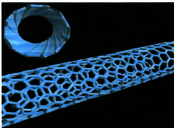
Σχήμα 2.18 Μονοφλοιικός νανοσωλήνας άνθρακα (SWCNT)
