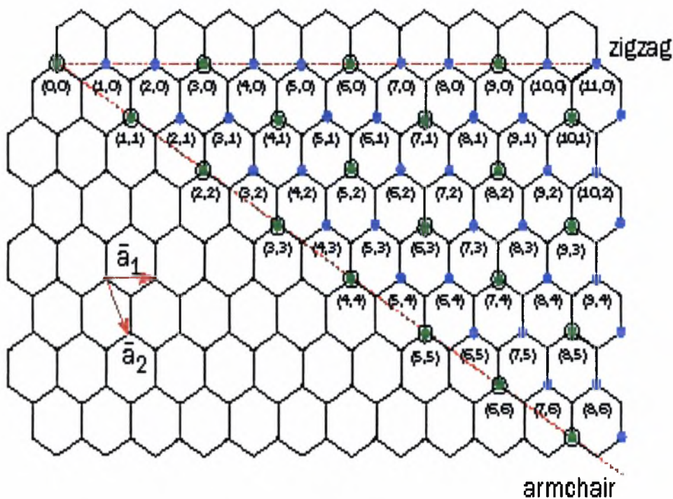
Σχήμα 2.21 Πιθανές δομές μονοφλοιικών νανοσωλήνων άνθρακα
