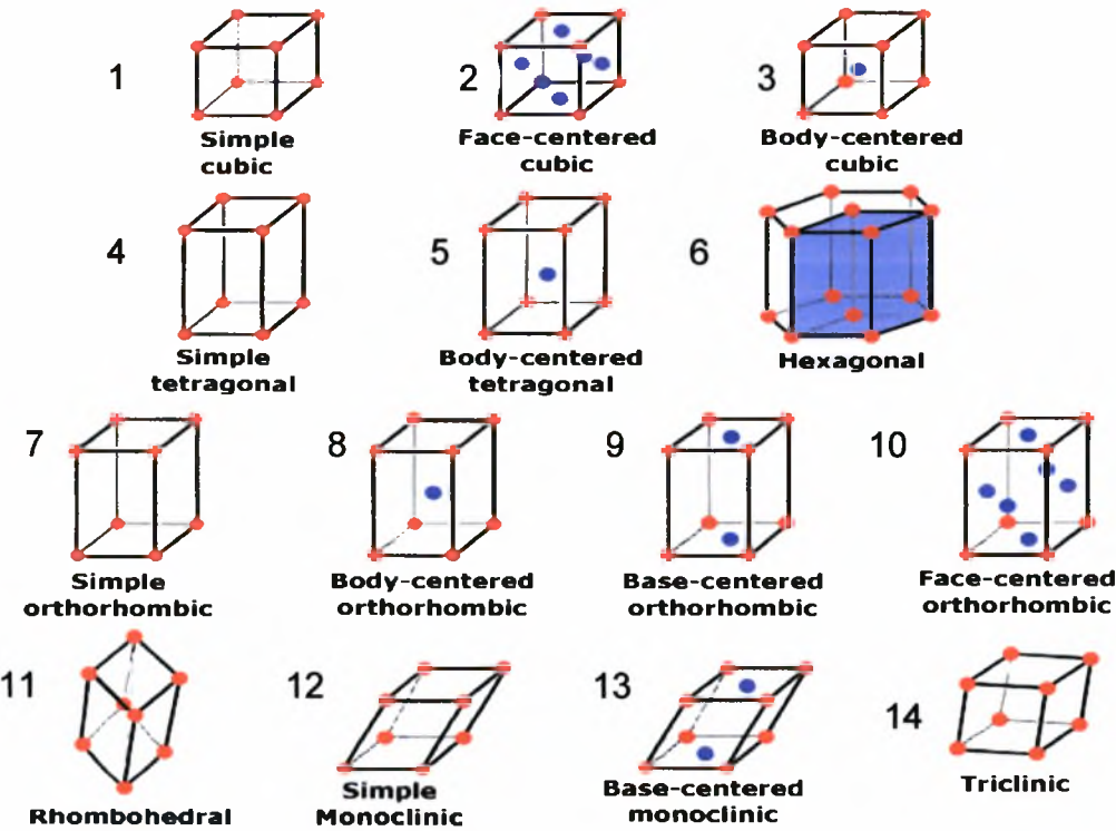
Σχήμα 2.1 Μορφές κρυσταλλικών πλεγμάτων
