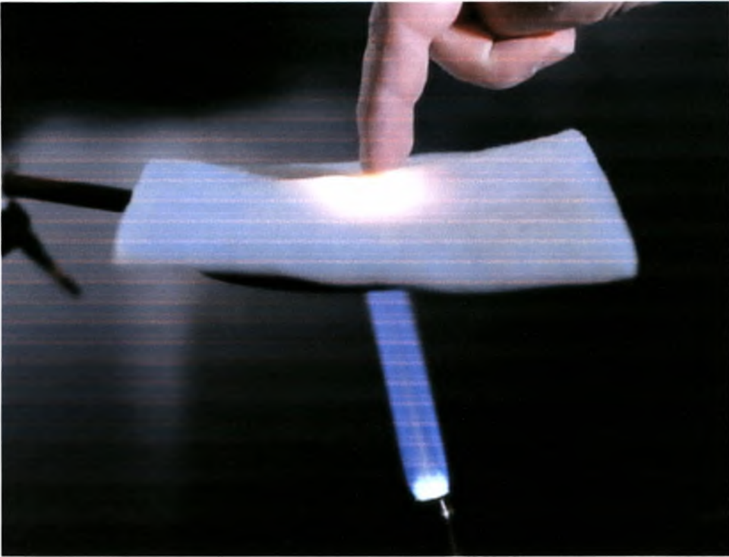
Σχήμα 3.13 Νανο-πορώδες μονωτική κουβέρτες: Πολύ χαμηλή θερμική αγωγιμότητα, αντοχή σε υψηλές θερμοκρασίες. Πυρίτιο αεροτζέλ με νανοσωματίδια σε συνδυασμό με ενίσχυση ινών, (Bakker, 2008).
