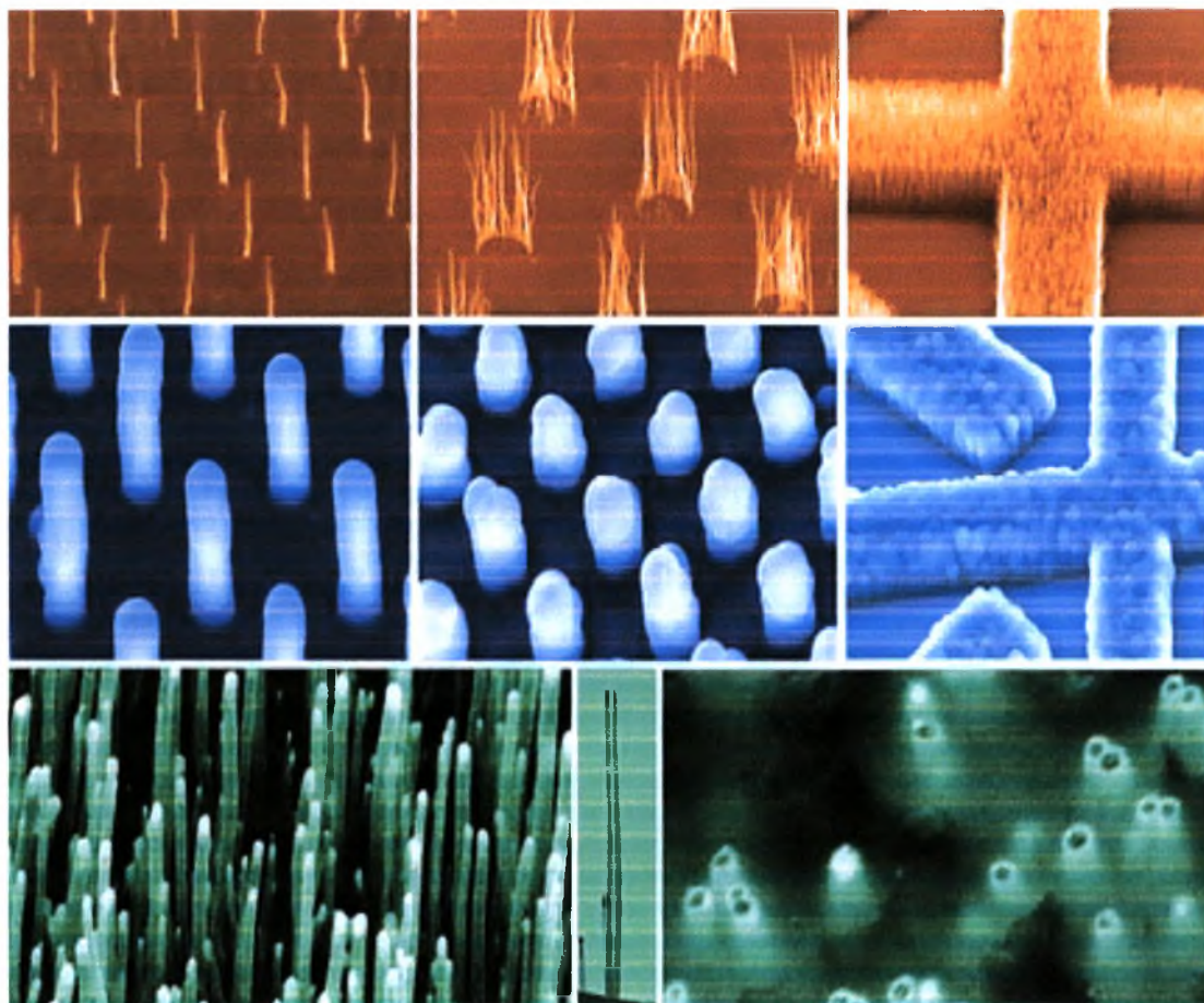
Σχήμα 2.14 Νανοσωλήνες (NASA, 2008)
