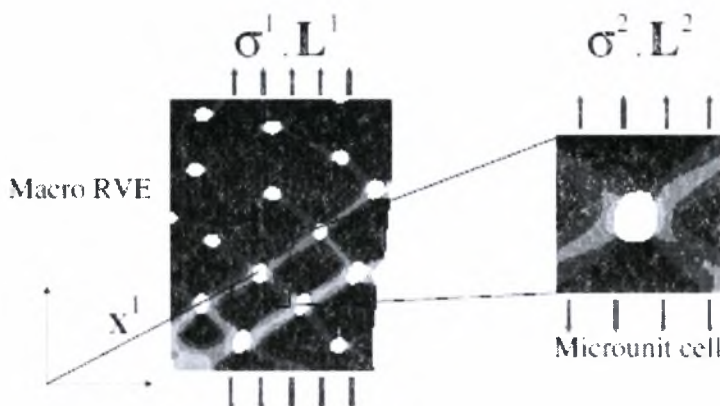
Σχήμα 4.5 Ένα μακρο αντιπροσωπευτικό στοιχείο όγκου RVE και μία κυψελίδα με τις αντίστοιχες πιέσεις τους και τους ρυθμούς των μέτρων παραμόρφωσης.
