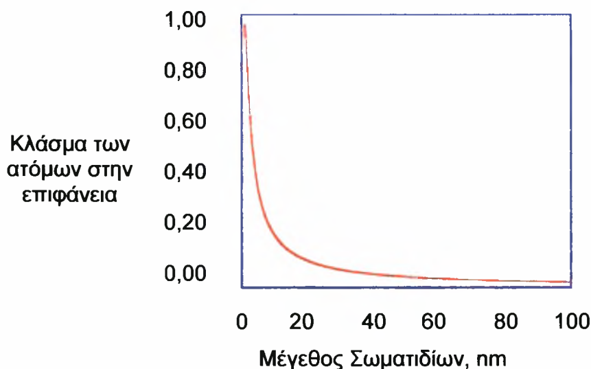
Σχήμα 2.10 Κλάσμα όγκου των ατόμων στην επιφάνεια ενός κυβοειδούς νανοςωματιδίου ως συνάρτηση του μεγέθους των νανοςωματιδίων, με βάση την εξίσωση (2,2).
