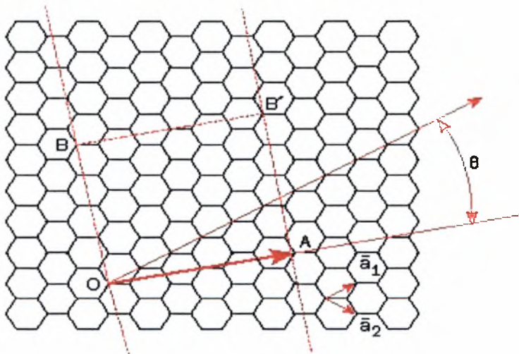
Σχήμα 2.19 Γραφитικό πλέγμα και απεικόνιση διανύσματος chiral
