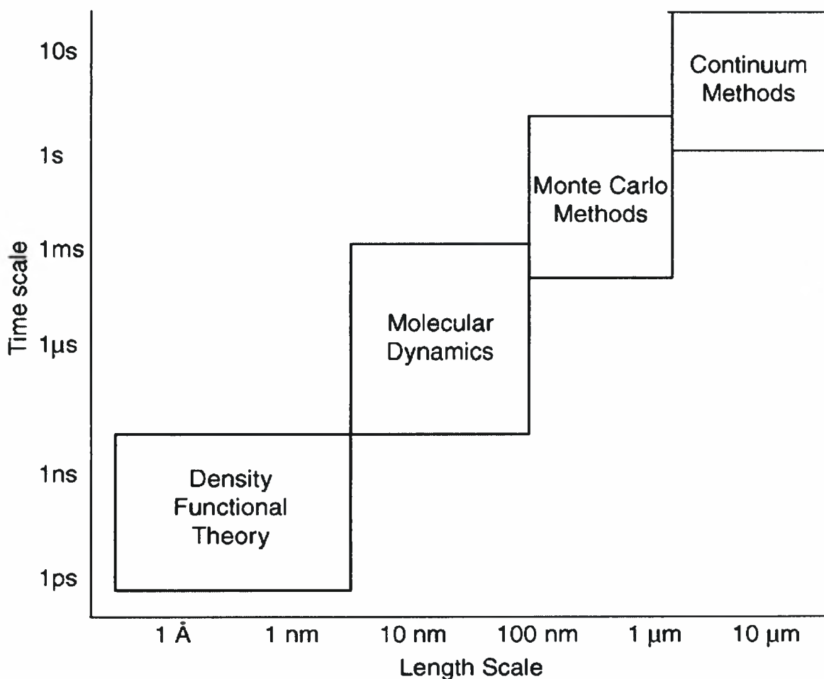
Σχήμα 4.2 Χαρακτηριστικές κλίμακες χρόνου και μήκους για διάφορες μεθόδους προσομοιώσεις υλικών, (Karakasidis Charitidis, 2007).
