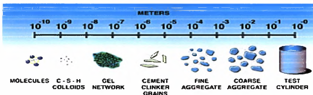
Σχήμα 3.2 Κλίμακες συστατικών σκυροδέματος
