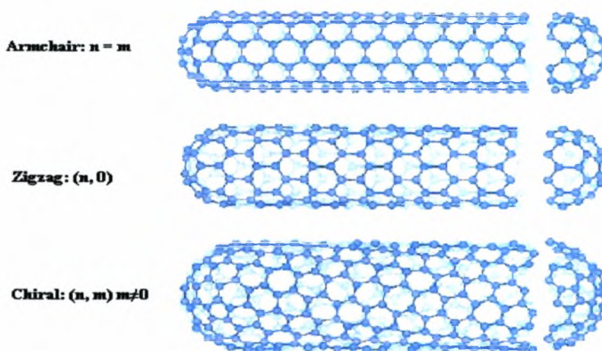
Σχήμα 2.20 Armchair, Zigzag και Chiral νανοσωλήνες άνθρακα
