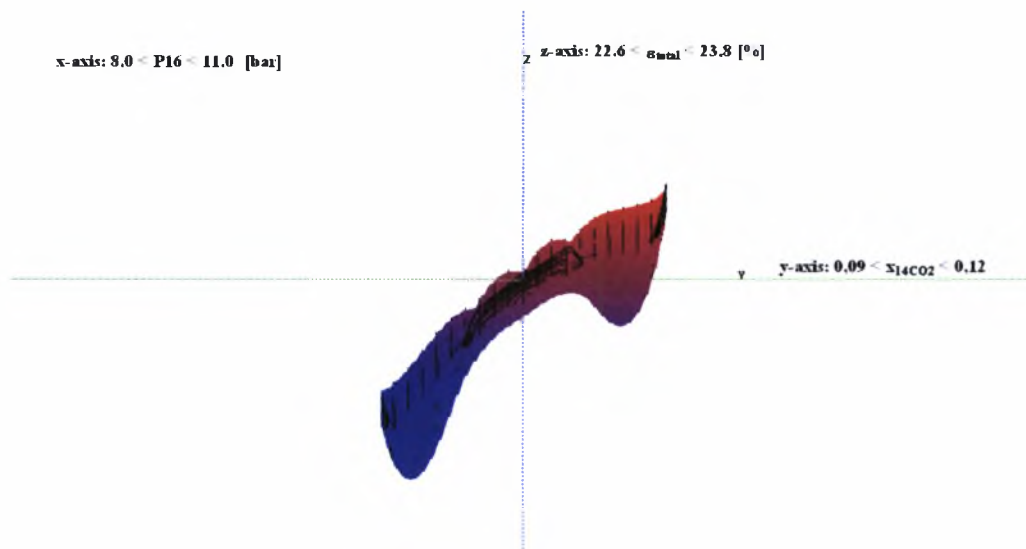
Σχήμα 5-11 (α), (β), (γ): Εξεργειακός βαθμός απόδοσης συστήματος σε σχέση με την πίεση P_{16} και την περιεκτικότητα X_{14CO_2} .
