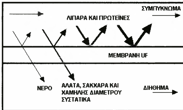
Σχήμα 2-1: Διαχωρισμός συστατικών γάλακτος και τυρόγαλου με τη χρήση μονάδων
