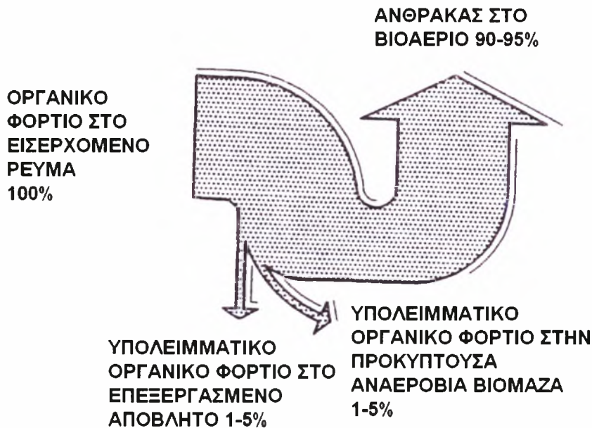
Σχήμα 2-2: Ισοζύγιο μετατροπής άνθρακα κατά την αερόβια και την αναερόβια επεξεργασία λυμάτων
