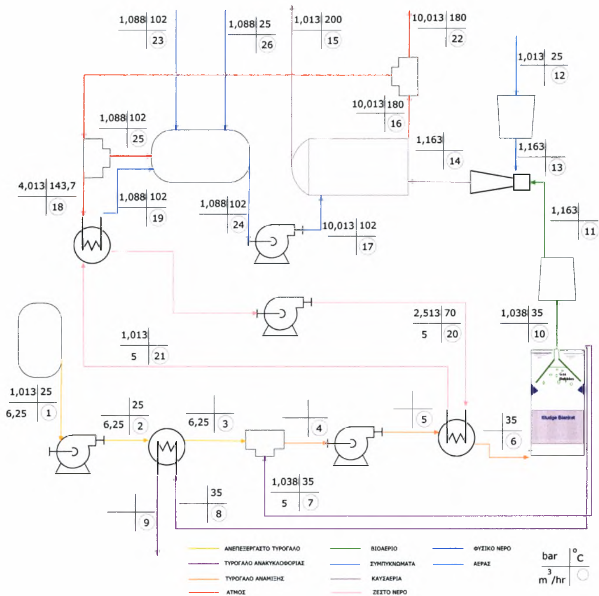
Σχήμα 3-2: Διάγραμμα ροής αναερόβιας επεξεργασίας τυρόγαλο
