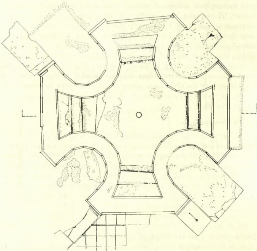
Εἰκ. 2. Κάτοψις τῆς κολυμβήθρας.
