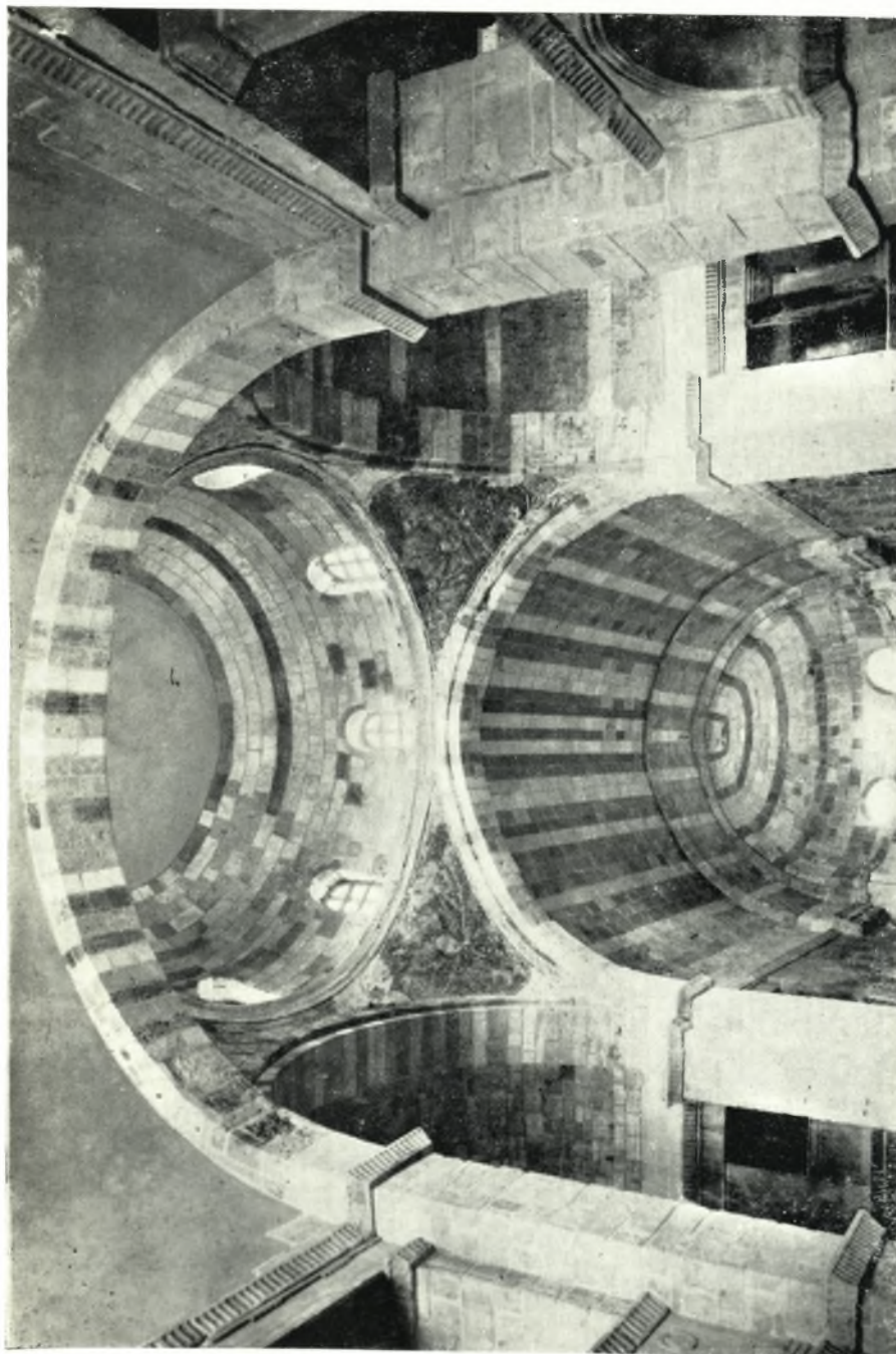
Ἐπιπέδους τοῦ προέλλου καὶ τοῦ θόλου τοῦ ἀνακτολικοῦ σκέλους τοῦ σταυροῦ τῆς Καταπολιανῆς μετὰ τὴν στερέωσιν καὶ τὸν καθαρισμόν των.
